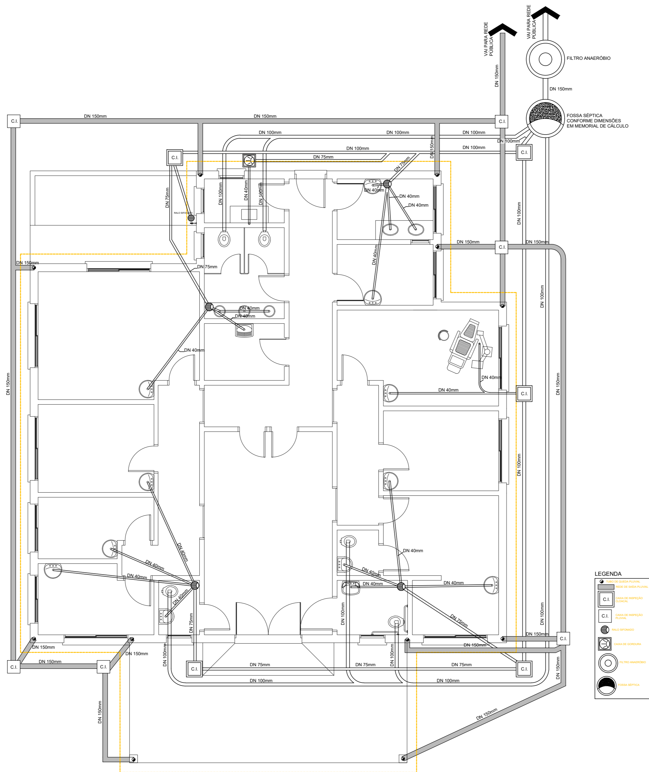
DISTRIBUIÇÃO REDE ESGOTO - EDIFICAÇÃO EXISTENTE Escala 1/50
