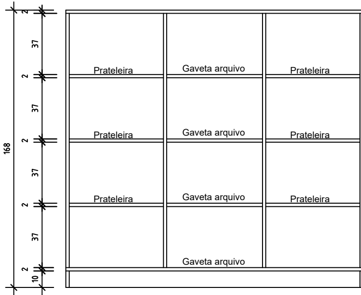
VISTA FRONTAL INTERNA ARMÁRIO
