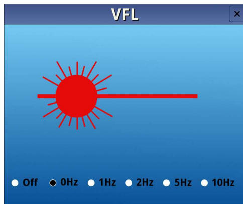
Na foto: O feixe do Localizador Visual de Falhas (VFL) ilumina curvas, emendas e falhas em fibras ópticas, com alcance efetivo de até 10 km.
