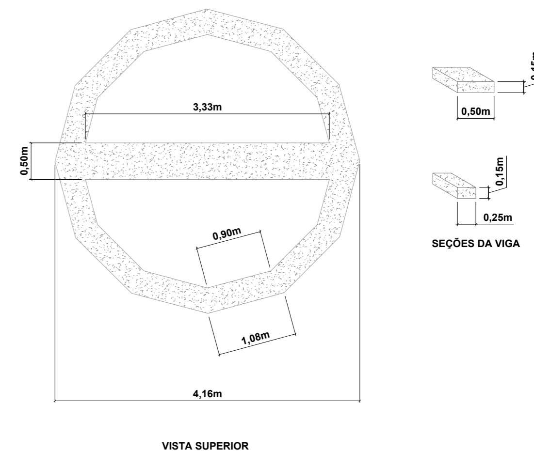
VIGA DE CONCRETO ARMADO ESCALA 1:50
