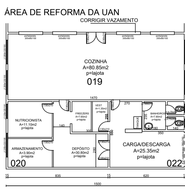
PLANTA BAIXA COZINHA E ARMAZENAMENTO
