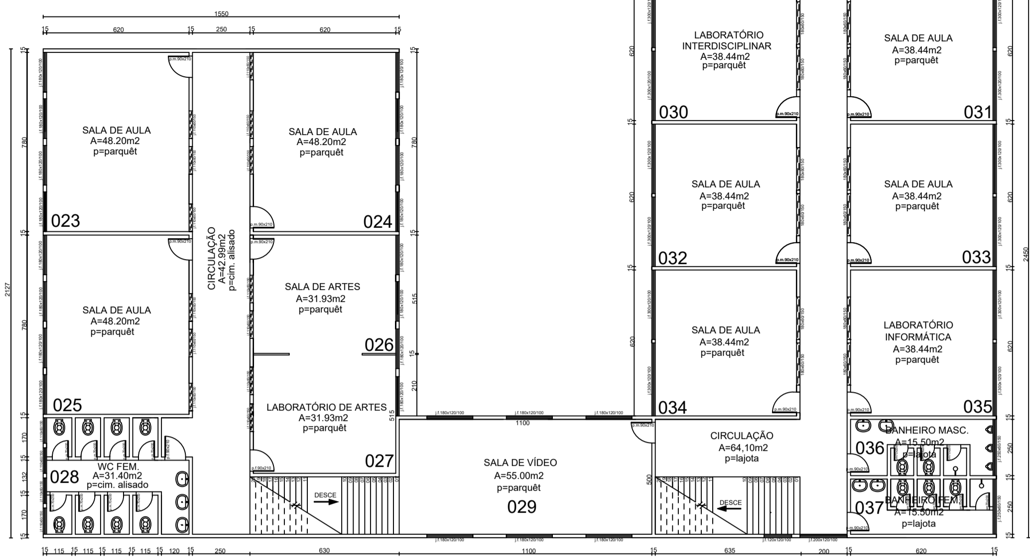
PLANTA BAIXA PAVIMENTO SUPERIOR A=755,50m 2
