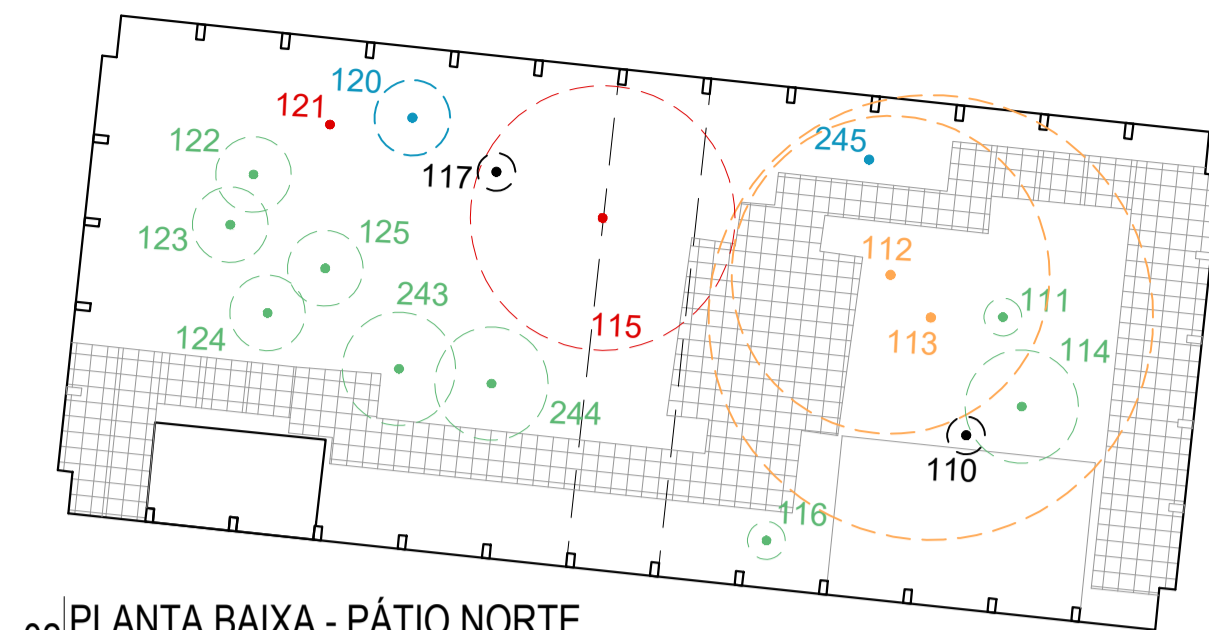
02 PLANTA BAIXA - PÁTIO NORTE ESC. 1:200
