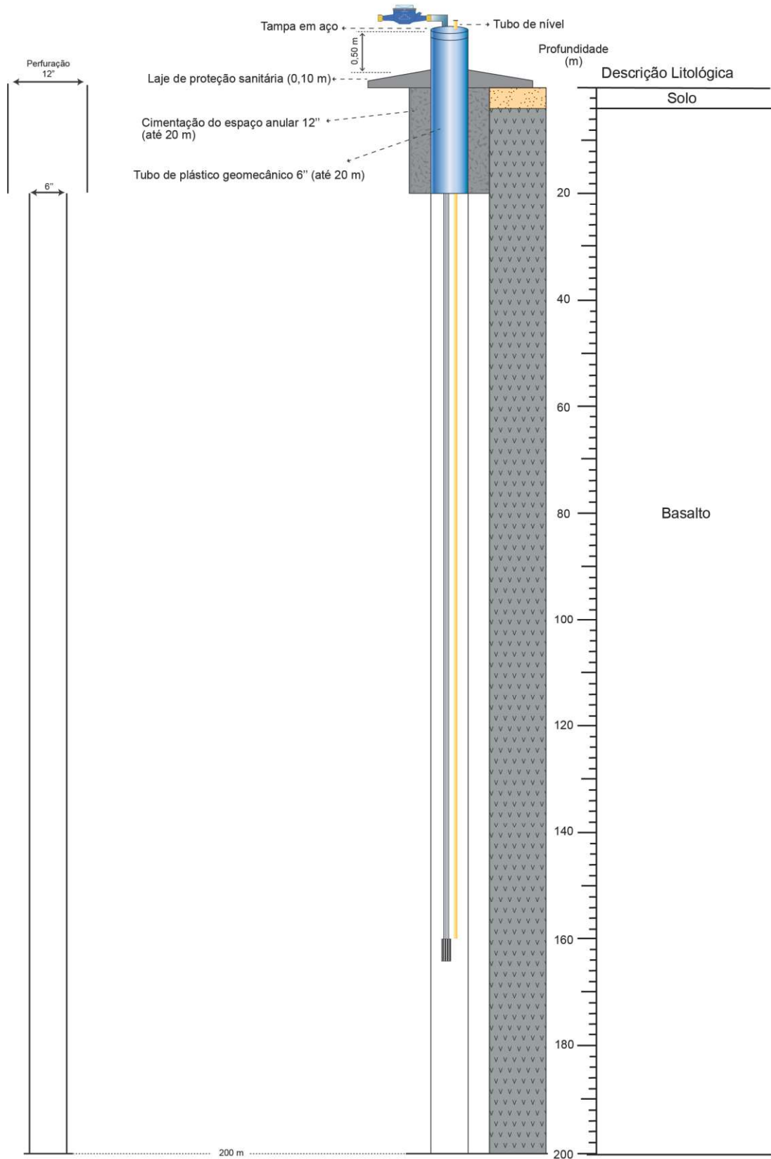
Figura 10. Perfil construtivo para um poço de 6" de diâmetro útil.
