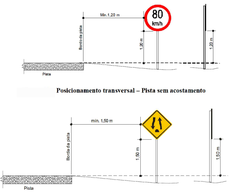
Figura 5 – Posicionamento dos sinais de regulamentação – Pista sem acostamento
