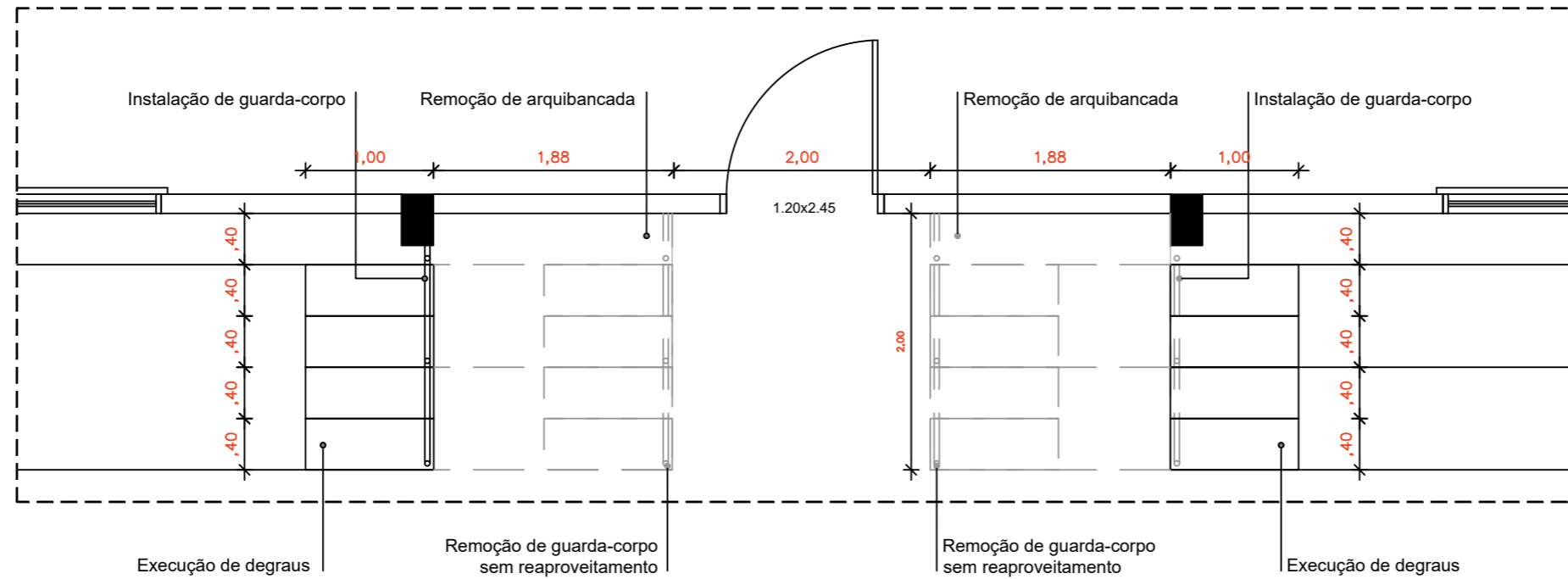
PLANTA-BAIXA DEMOLIR/CONSTRUIR
