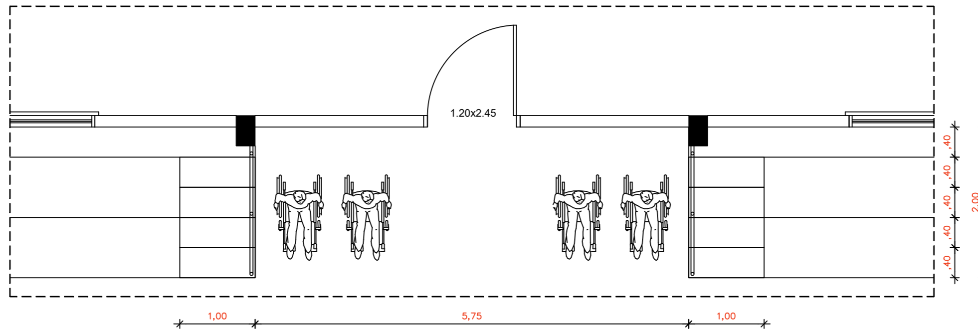
PLANTA-BAIXA DEFINITIVA
