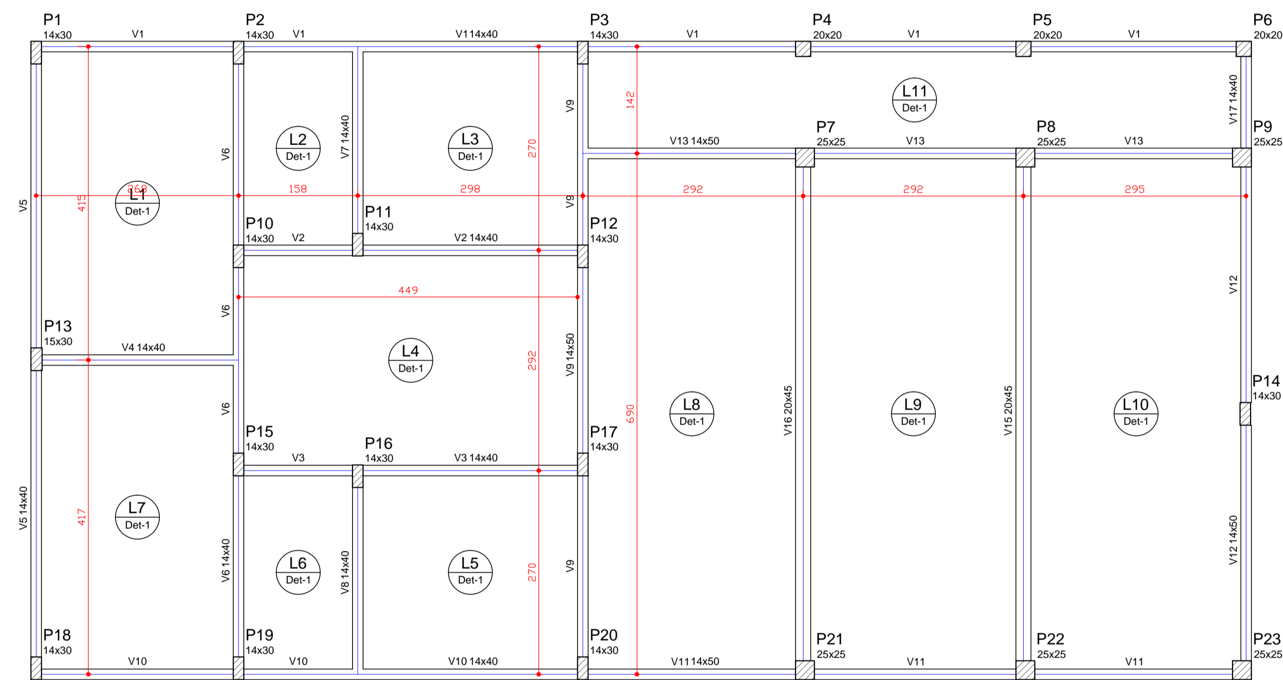
Forma do pavimento LAJE 1 escala 1:50
