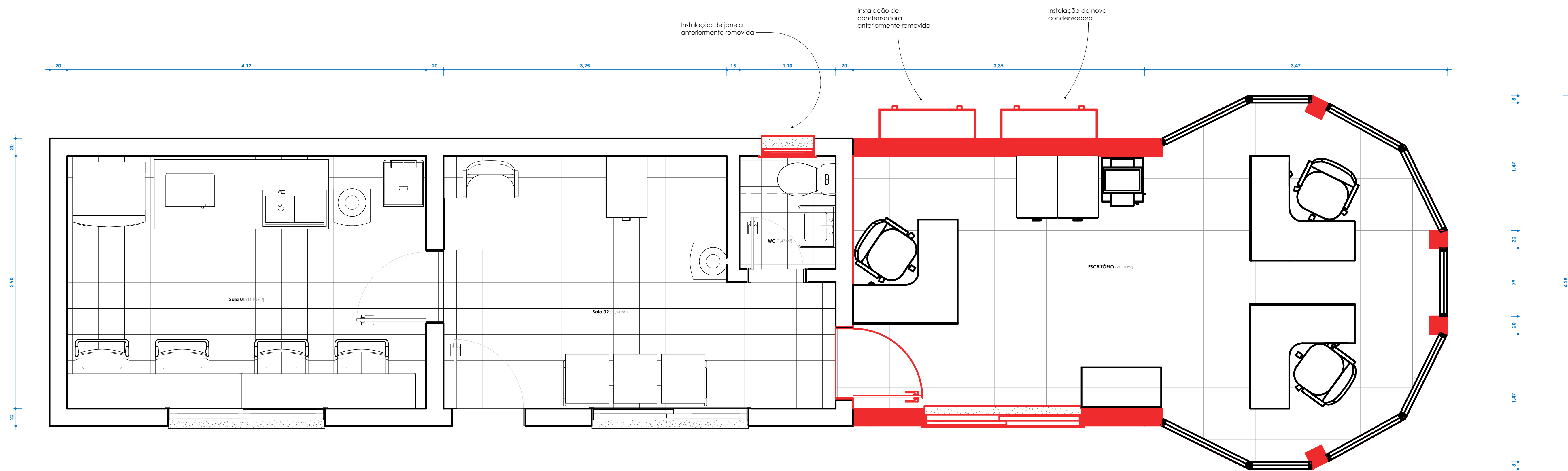
2 Térreo - Projeto Arquitetônico - A Construir 1 : 25
