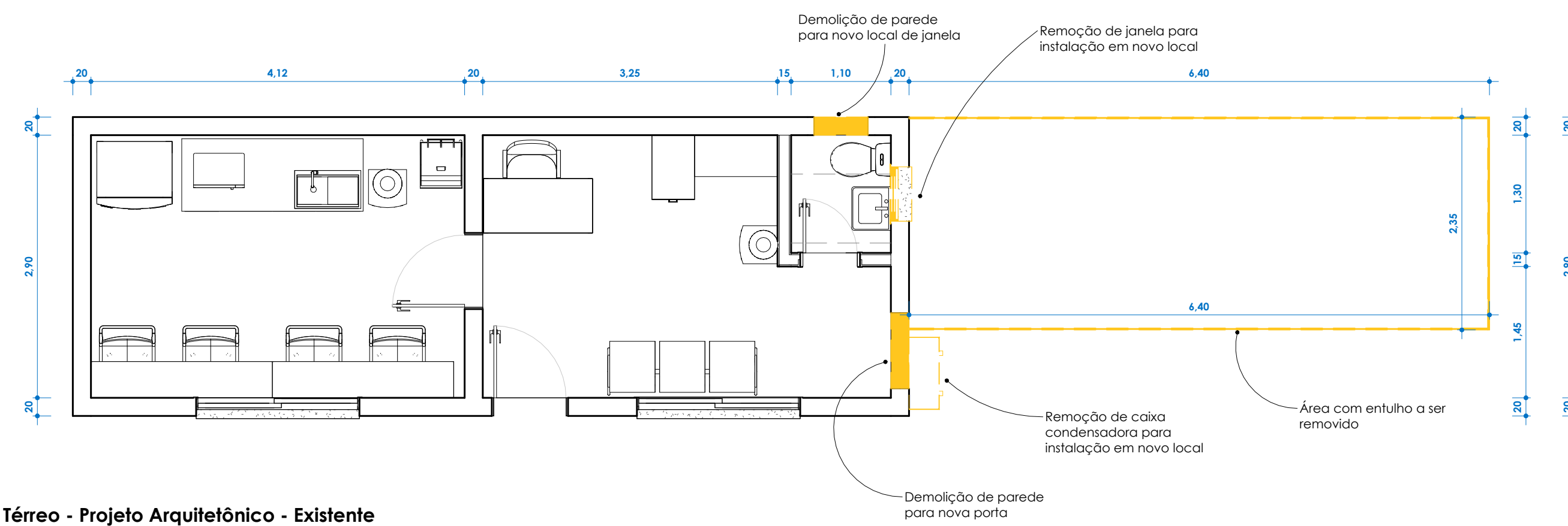
1 Térreo - Projeto Arquitetônico - Existente 1 : 50
