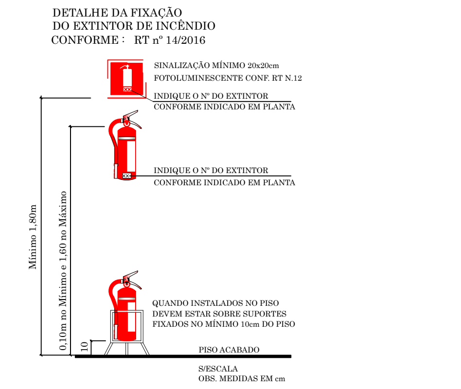
DETALHE 01 INSTALAÇÃO DE SINALIZAÇÃO
