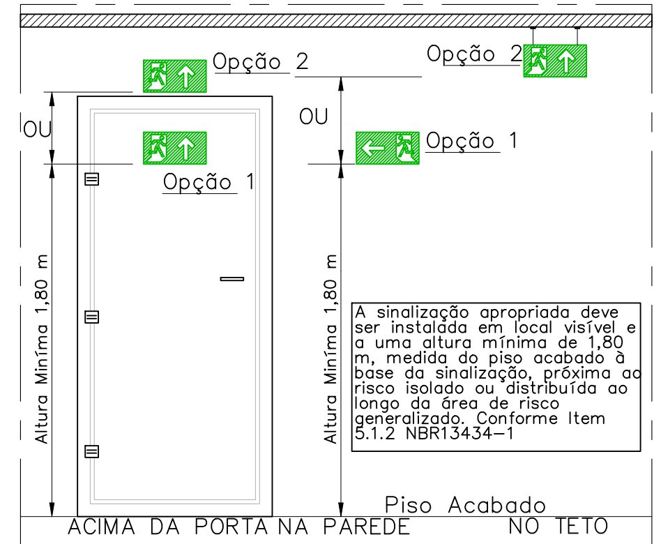
DETALHE 01 INSTALAÇÃO DE SINALIZAÇÃO
