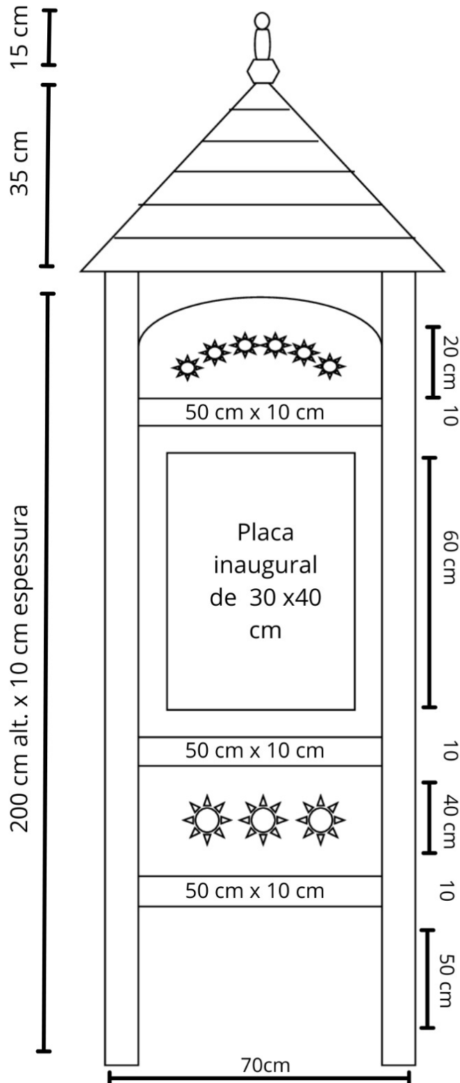
Figura 15 - Desenho e dimensões do Portal de Madeira.
