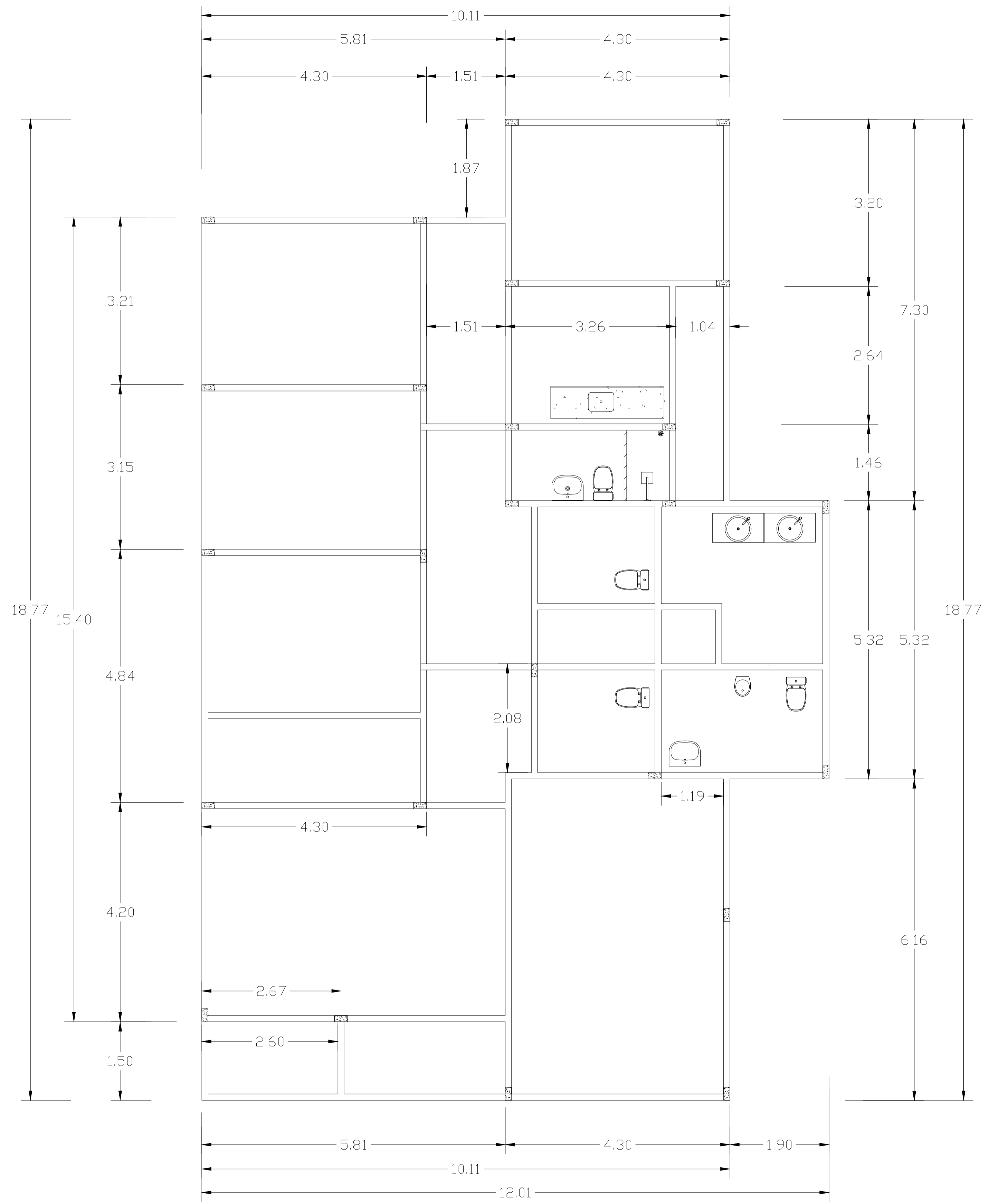
PILARES / VIGAS DE CINTAMENTO
