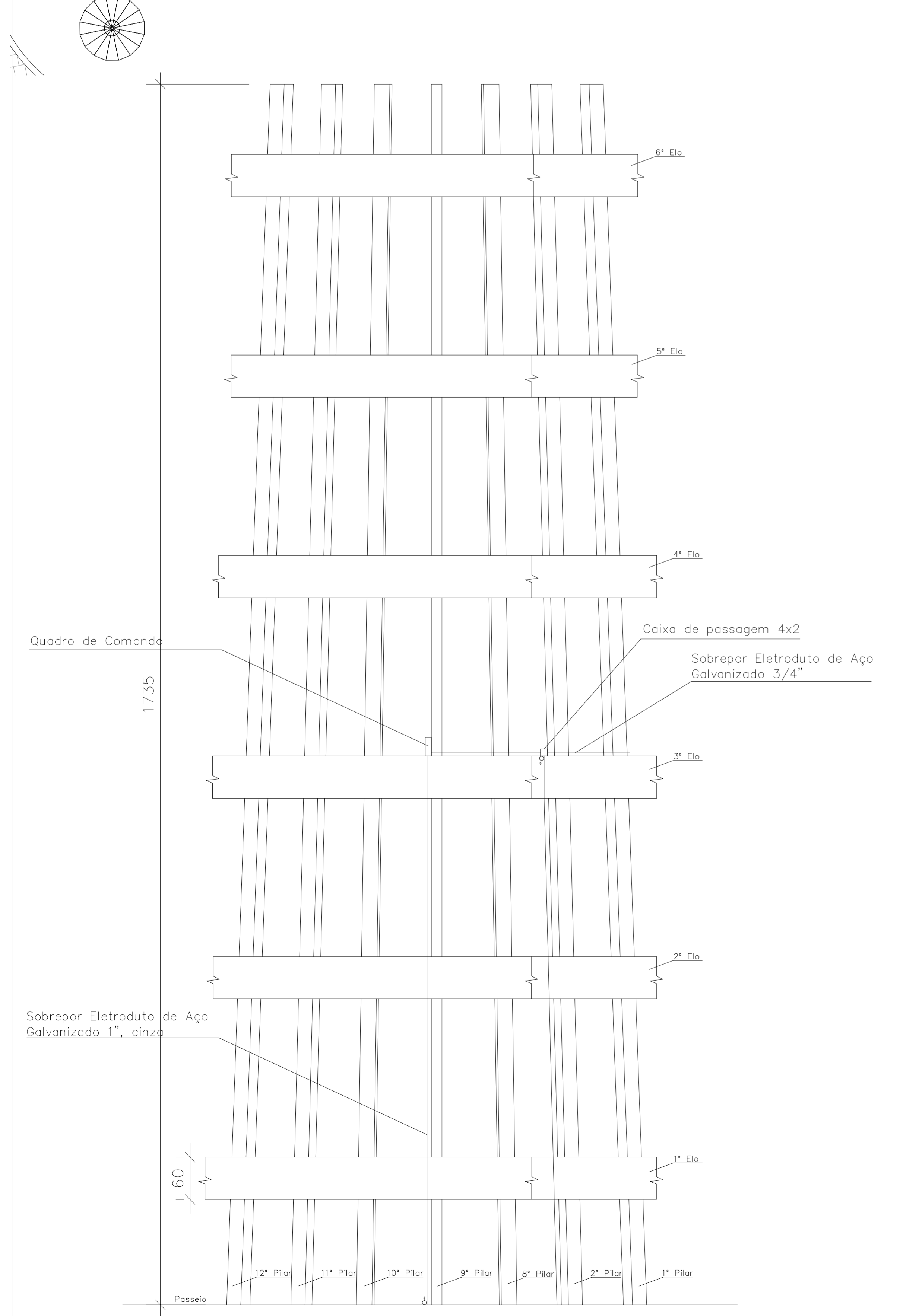
Corte S/Escala
