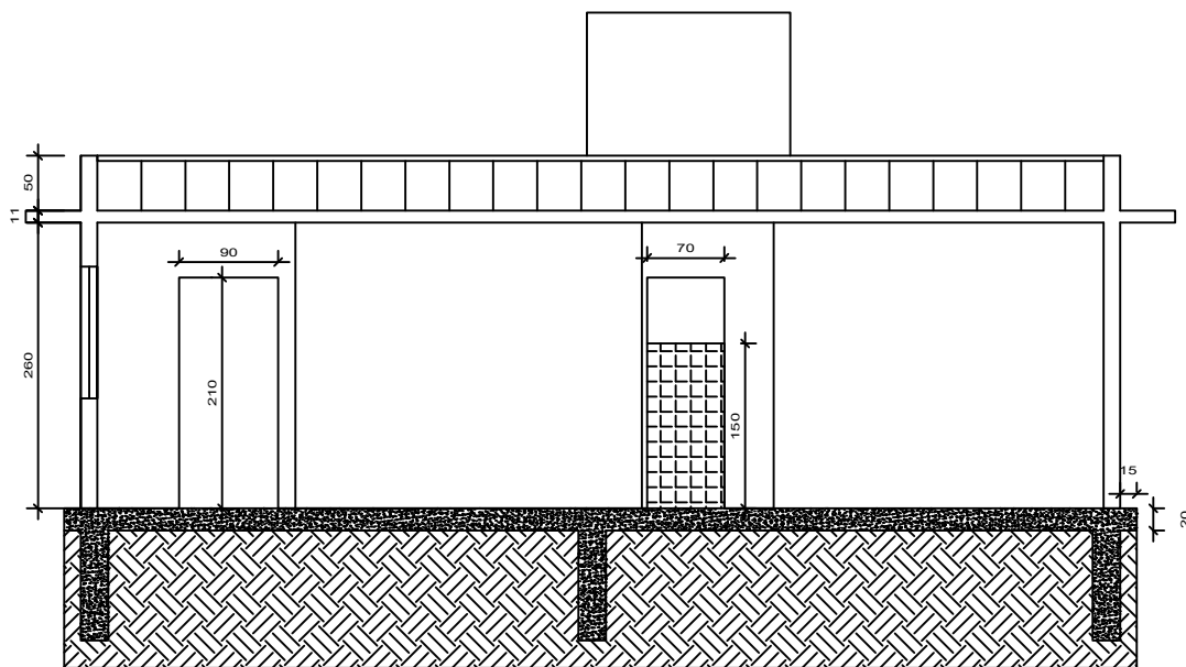
CORTE BB
