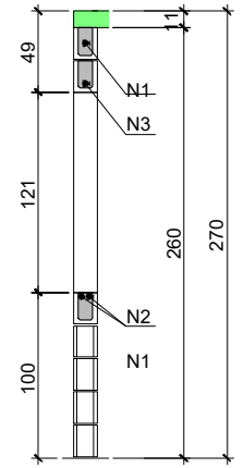
Corte A-A
