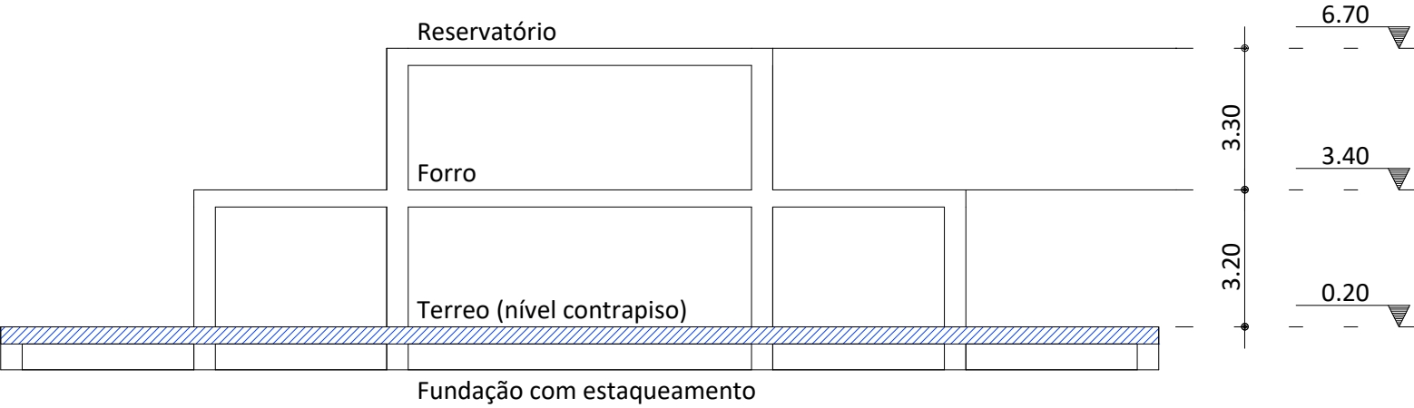
Corte Esquemático Estrutural
