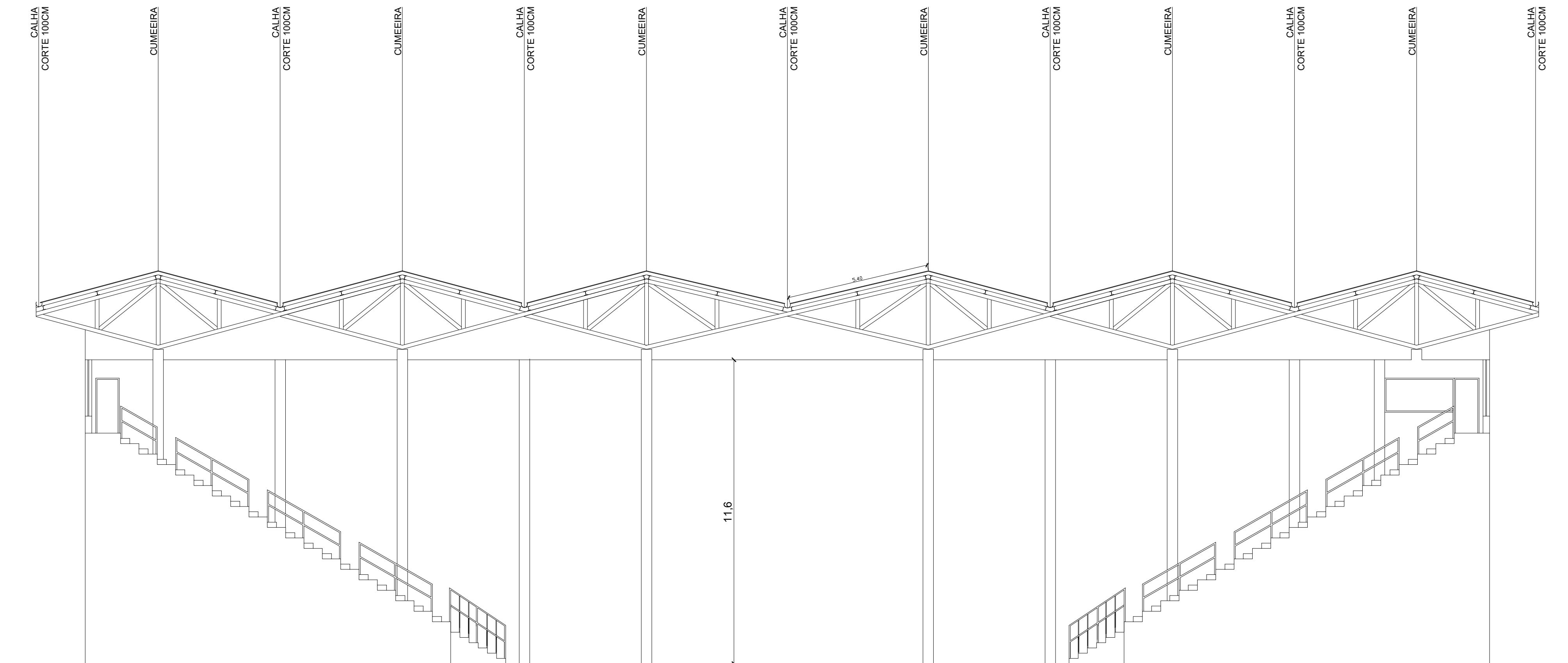
CORTE ESQUEMÁTICO - TELHADO GINÁSIO Área de telhado: 3.434,40m² esc.: S/ESC
