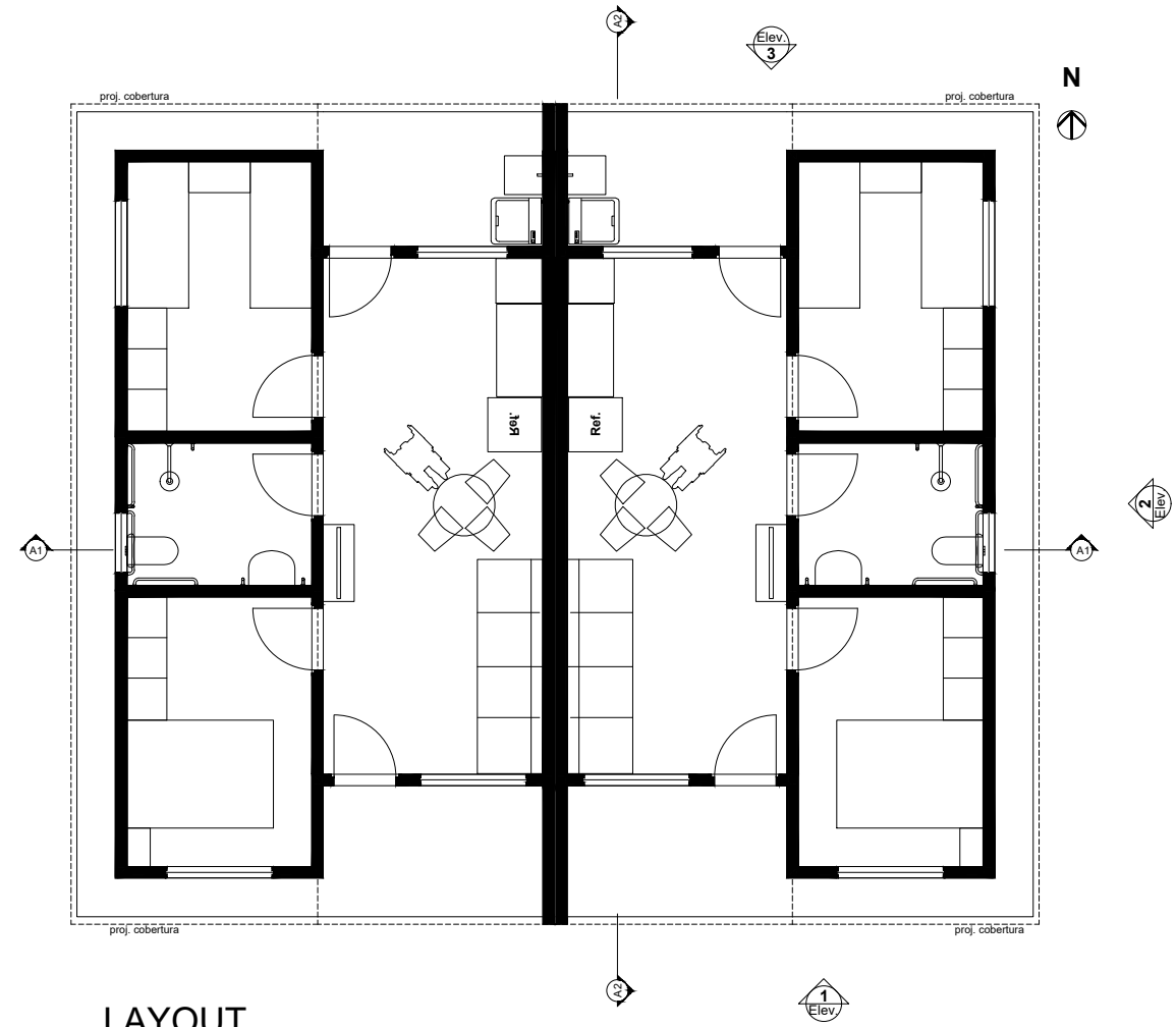
LAYOUT SEM ESCALA
