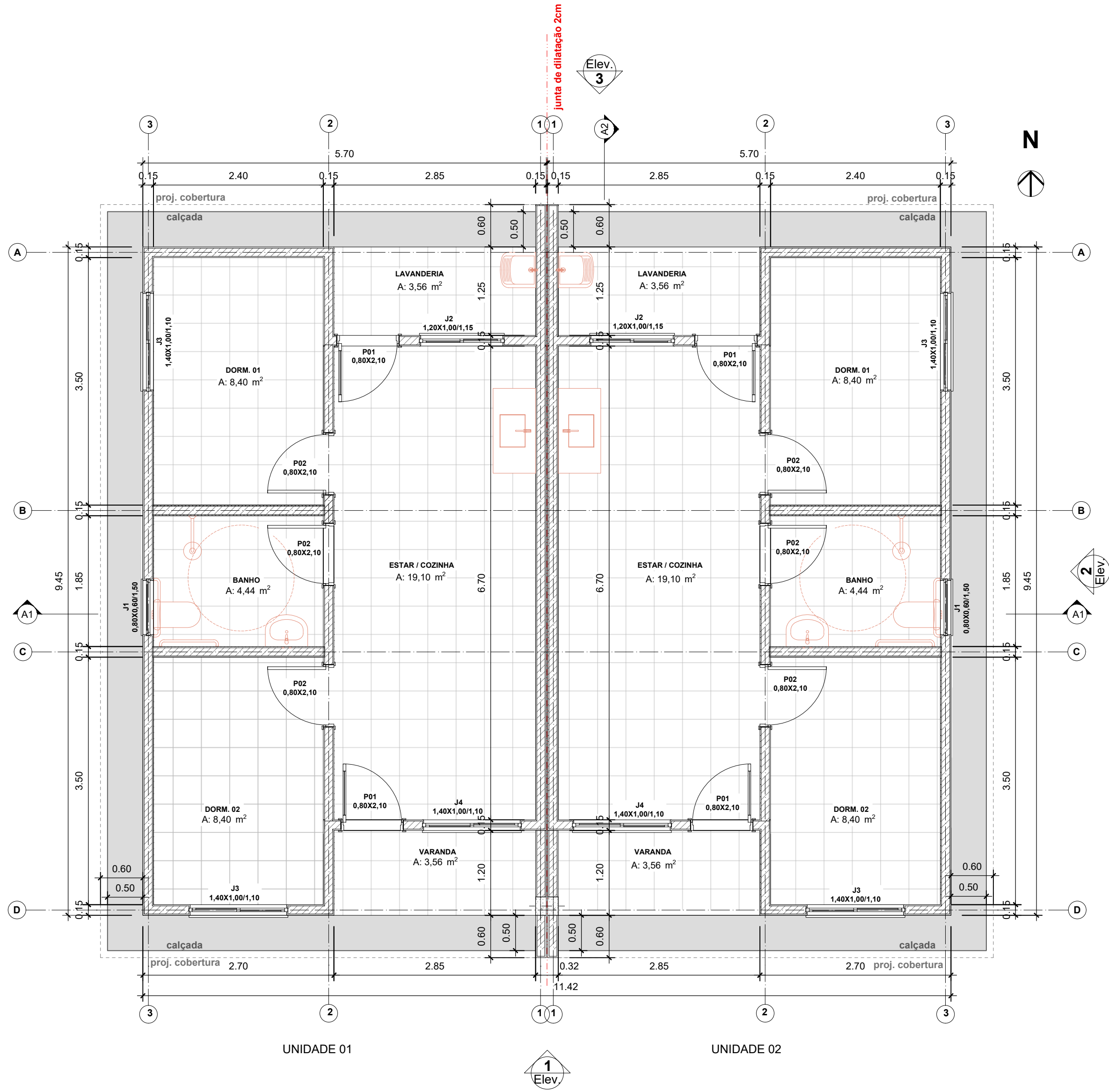
PLANTA-BAIXA ÁREA POR UNIDADE: 54,04m² ÁREA TOTAL: 108,08m² ESCALA 1:50
