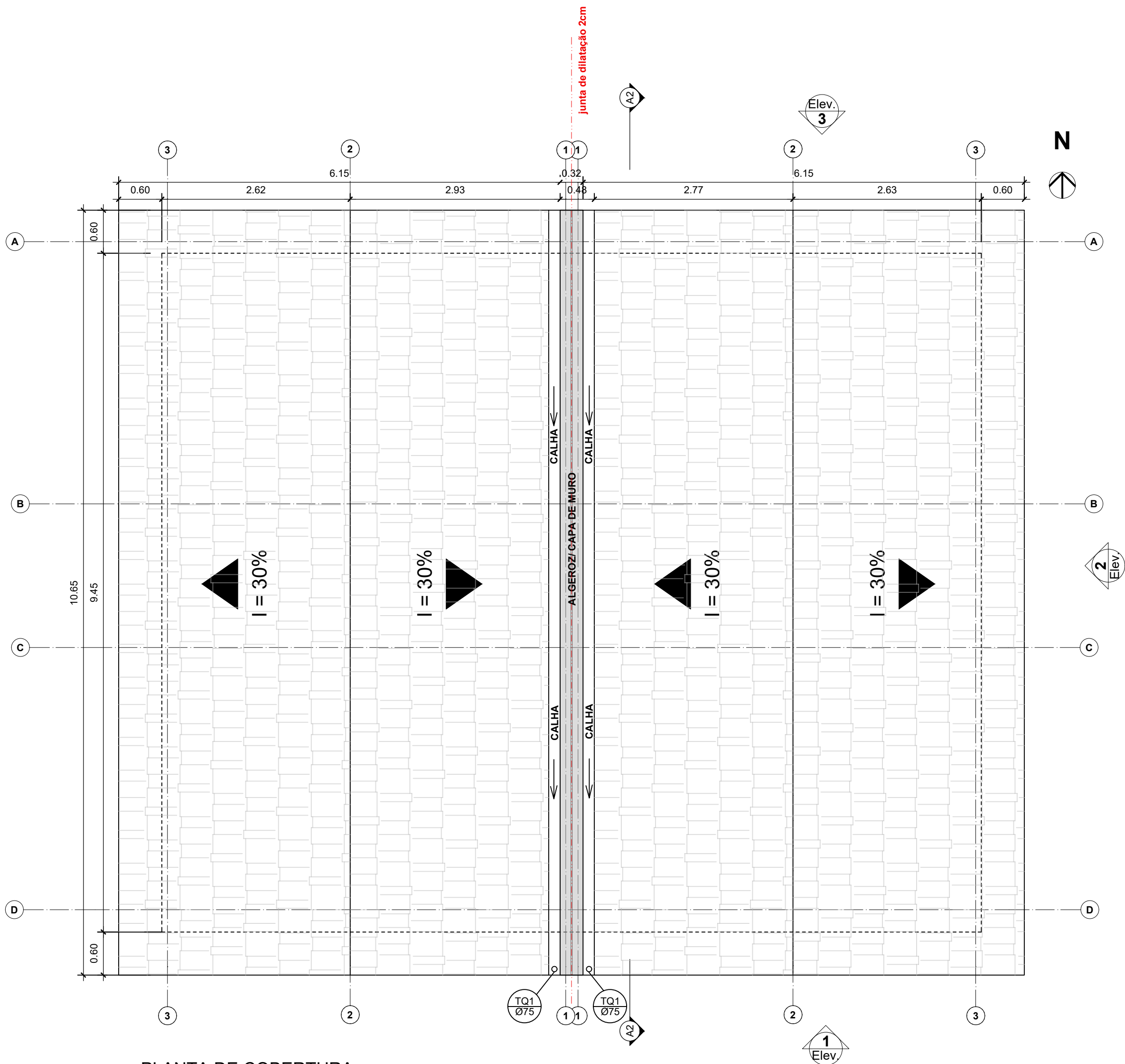
PLANTA DE COBERTURA ESCALA 1:50
