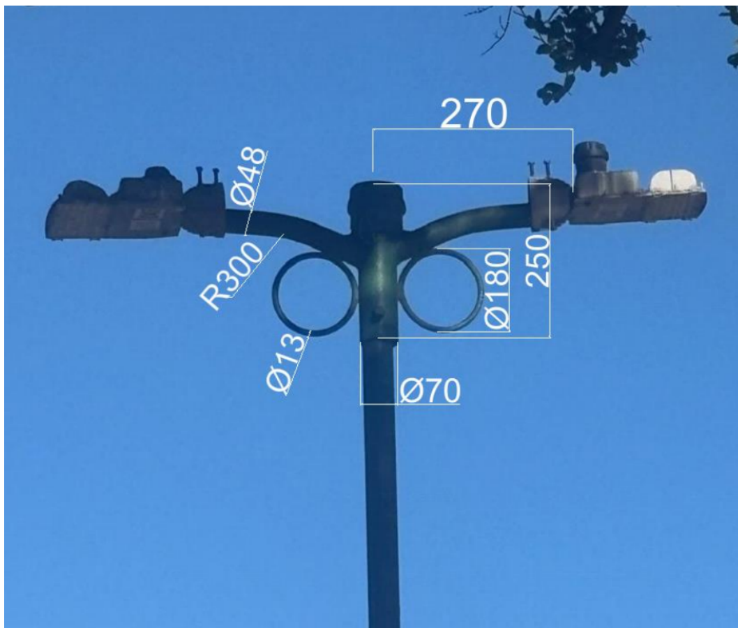
Figura 1: Dimensões do núcleo para 02 (duas) luminárias
