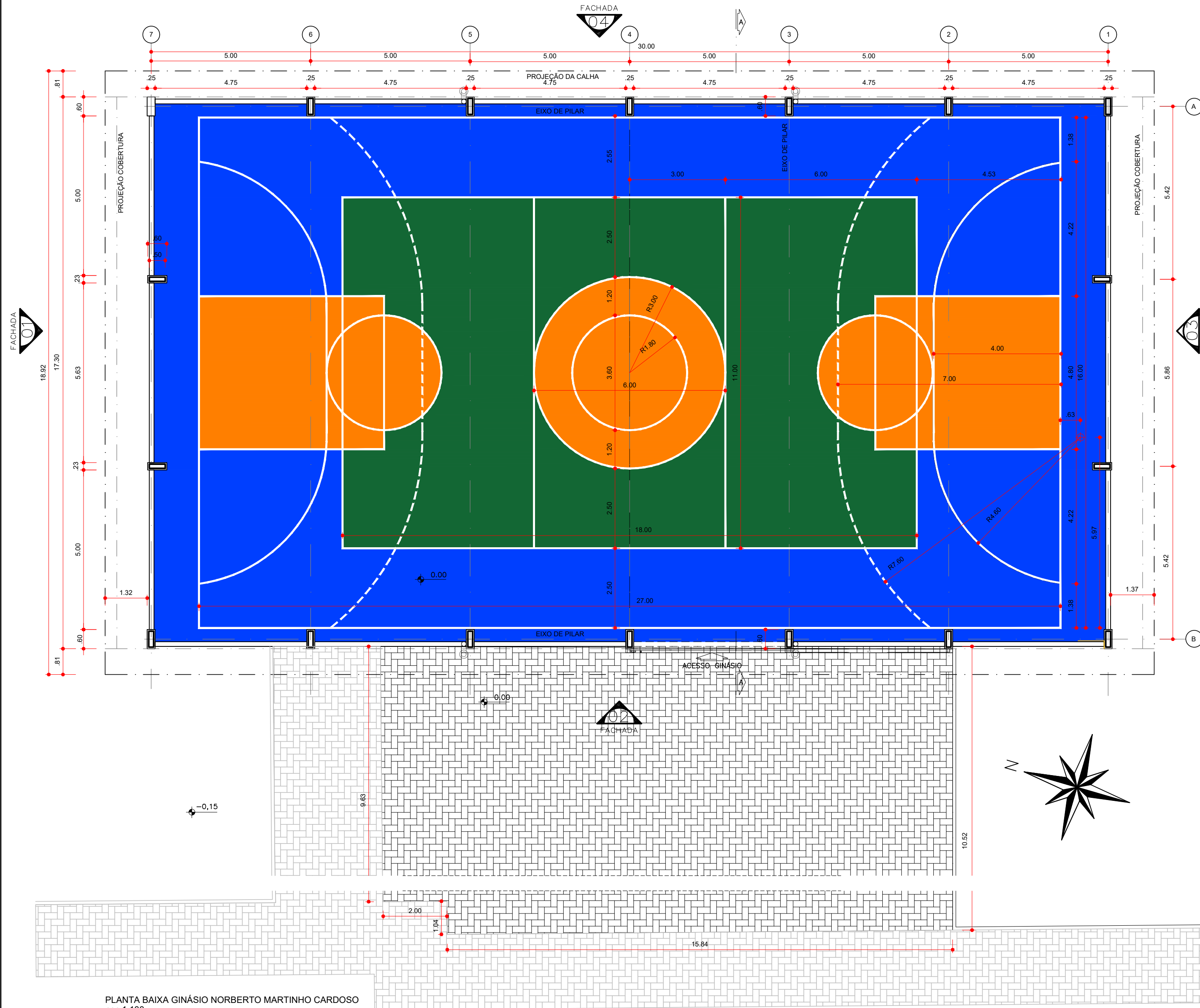
PLANTA BAIXA GINÁSIO NORBERTO MARTINHO CARDOSO esc 1:100
