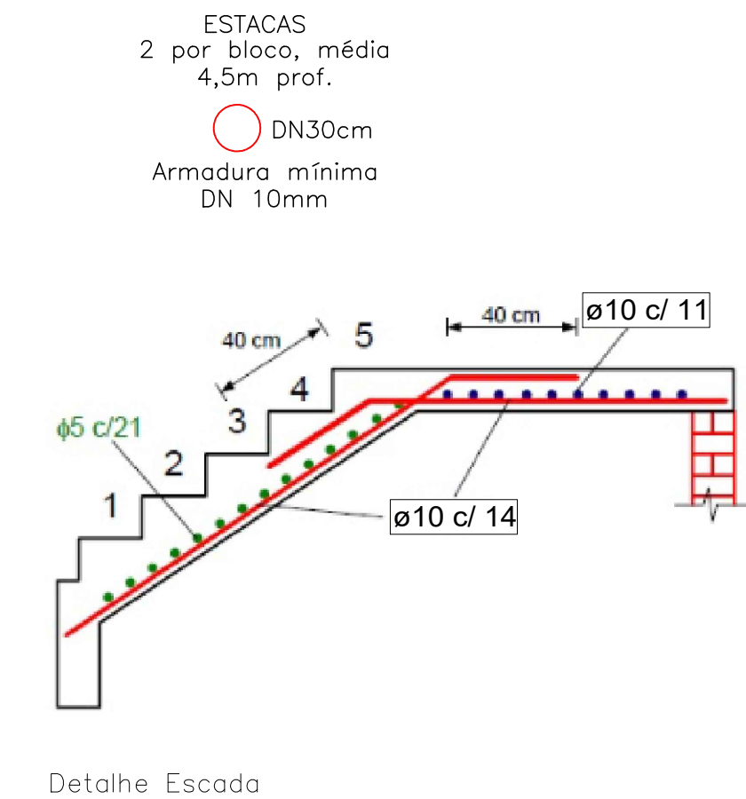
Detalhe Escada
