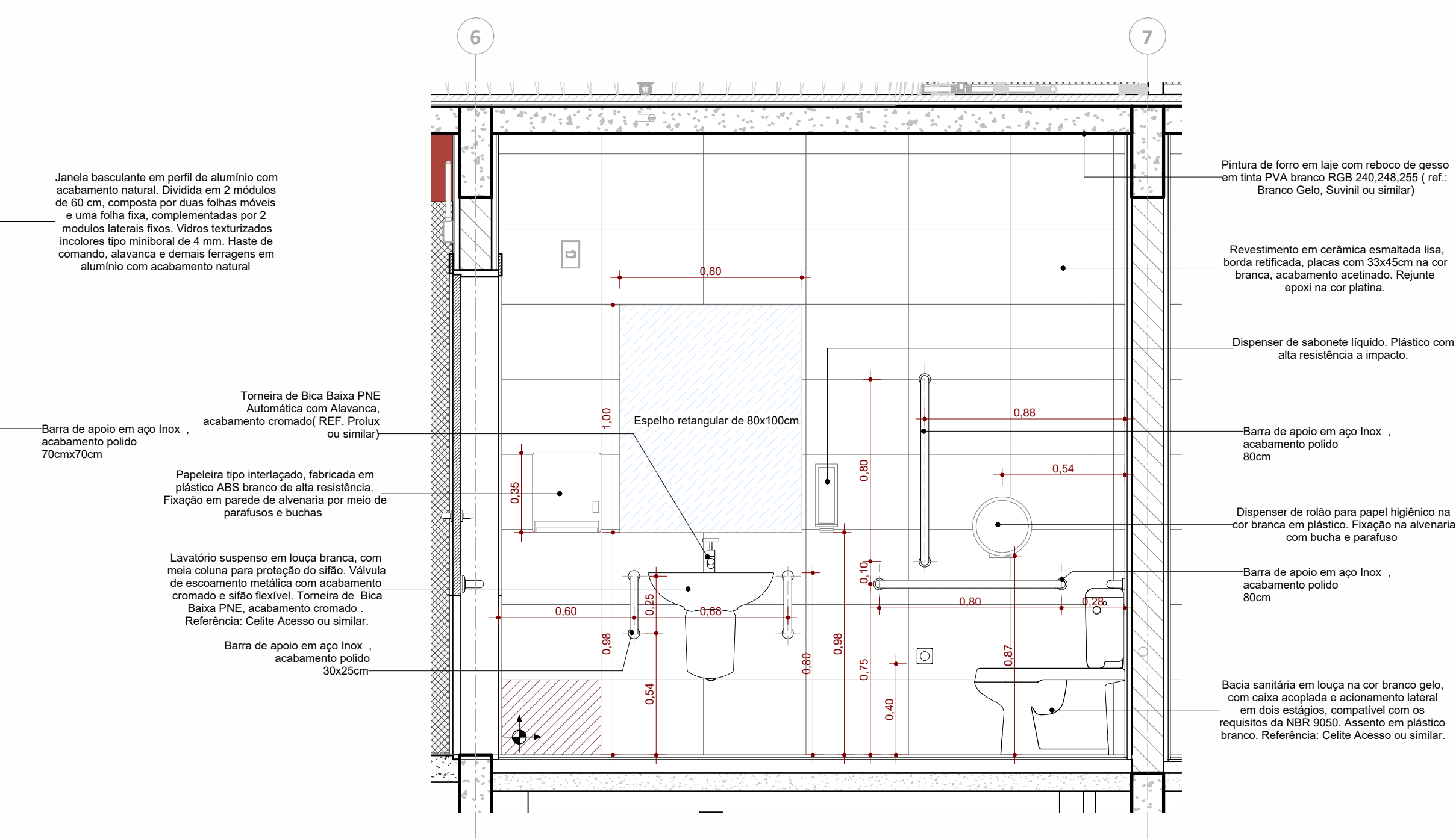
VISTA 12
