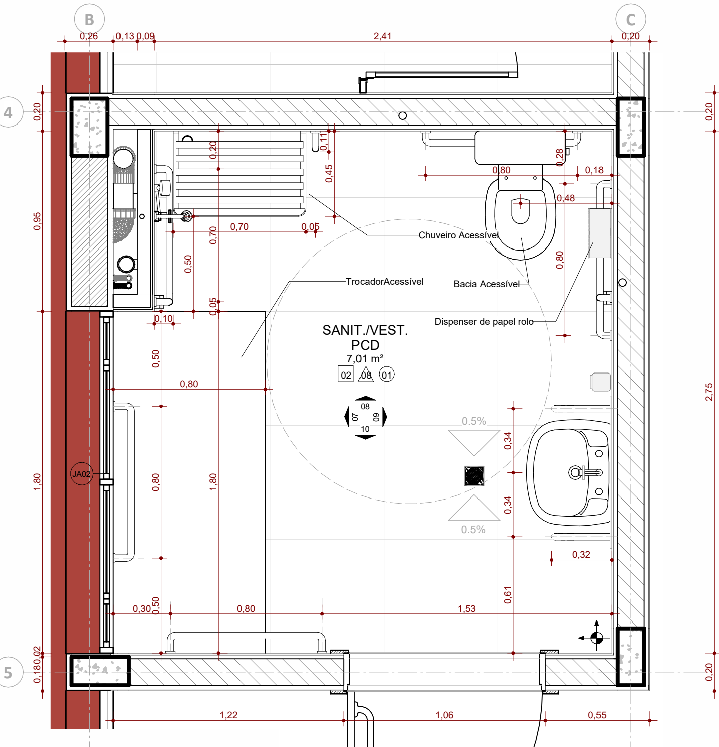
Detalhe Vestiário Masc PNE
