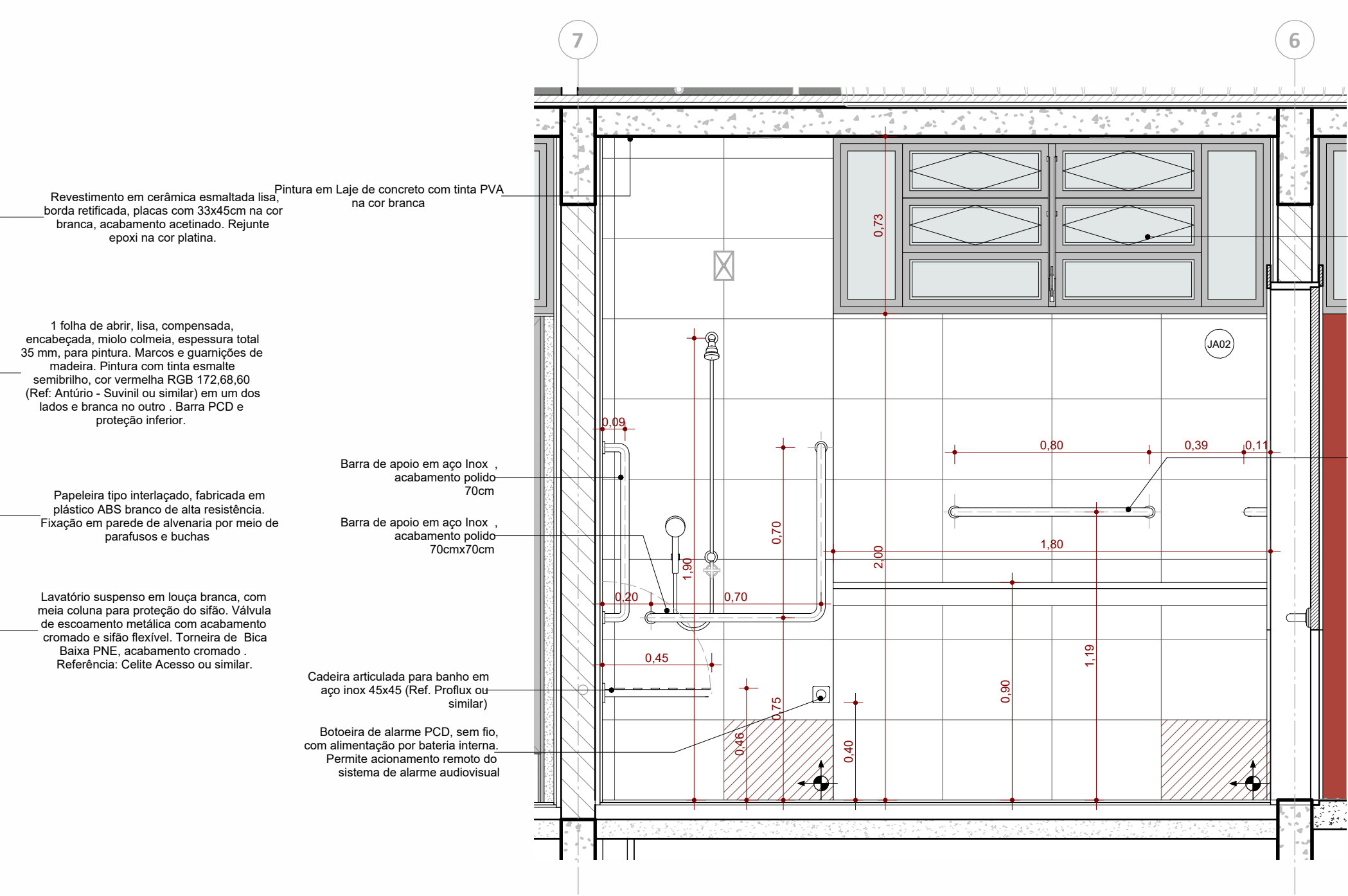
VISTA 11
