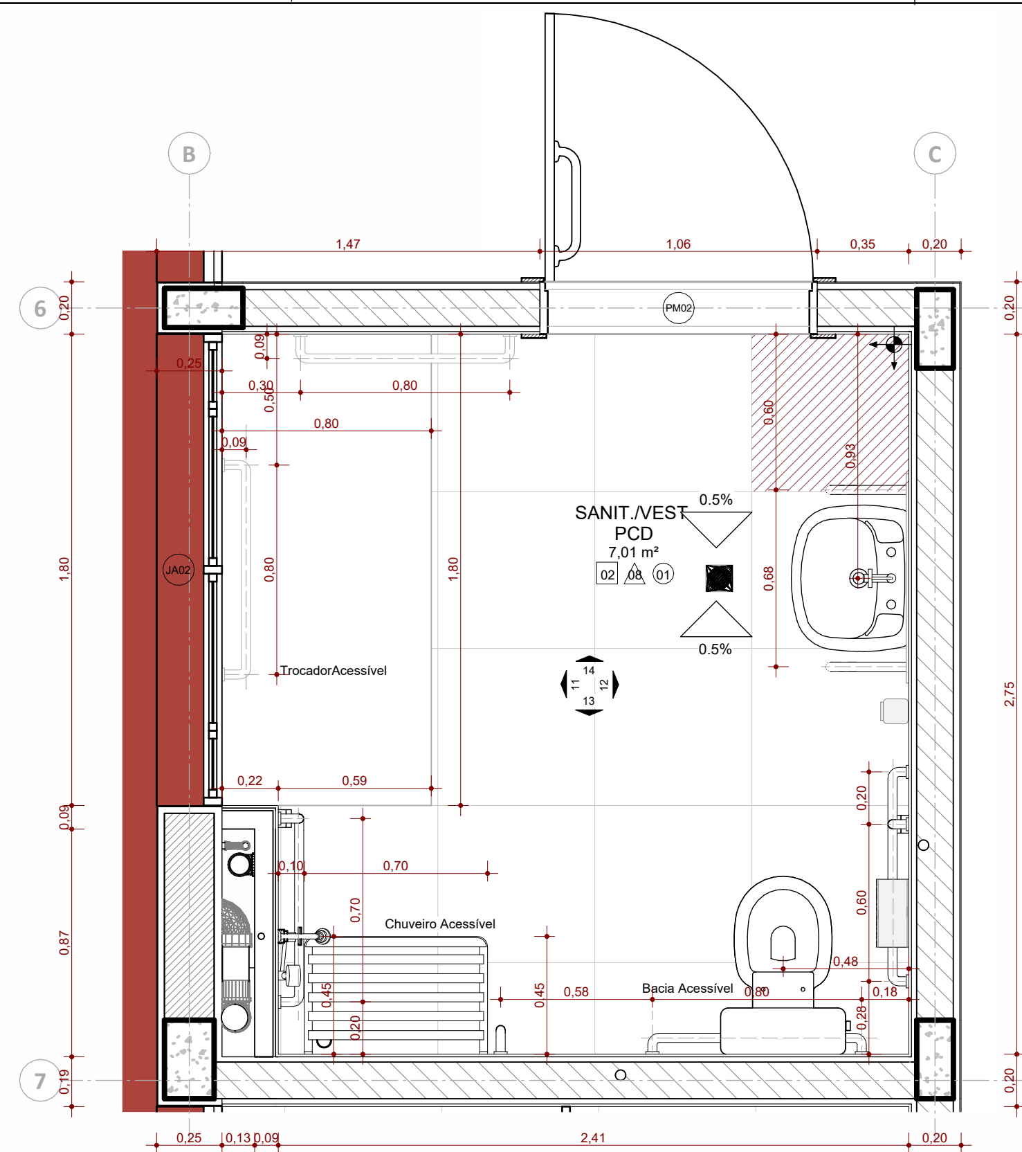
DETALHE - VESTIÁRIO PNE FEM.
