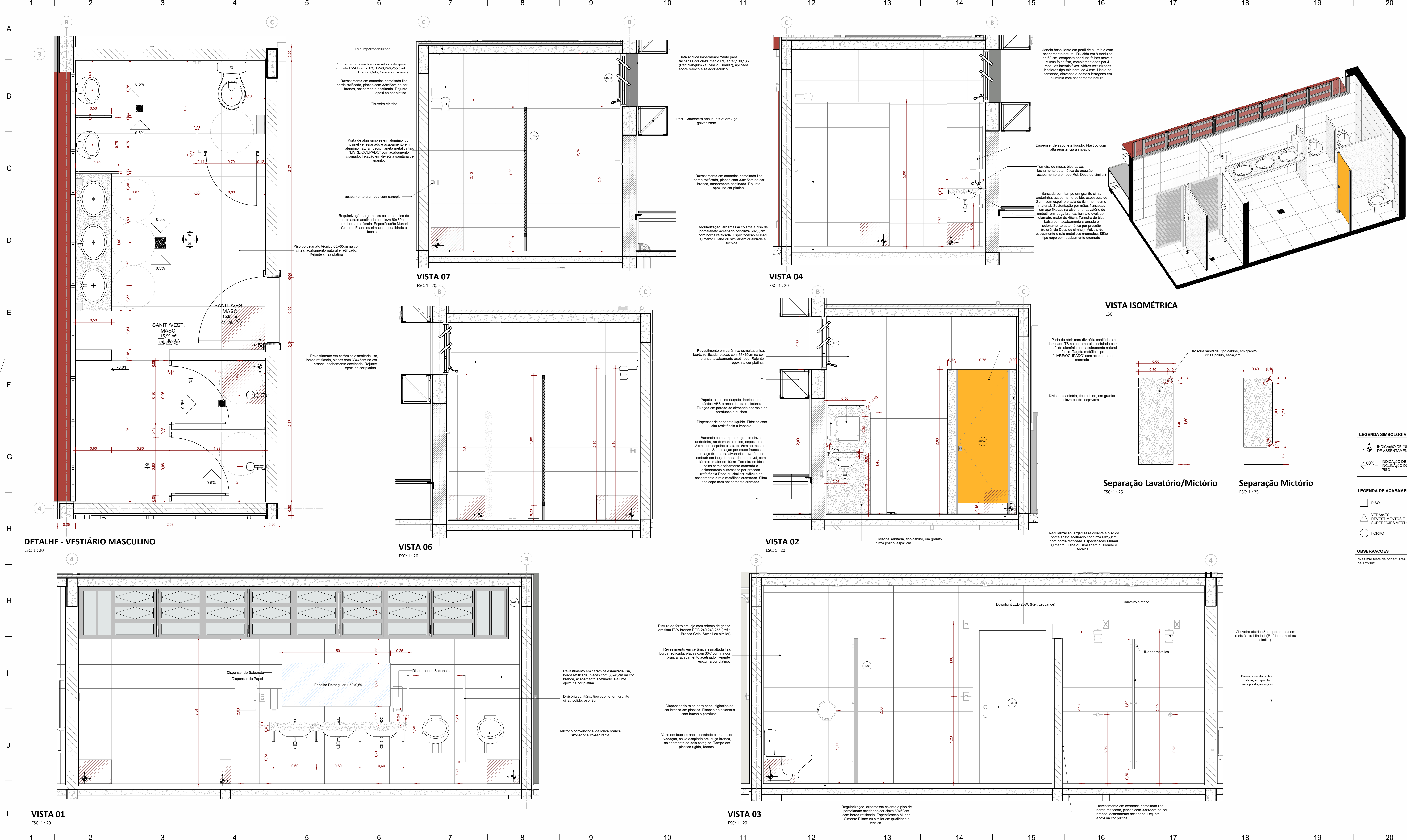
Croqui de Referência - Vest Masc ESC: 1 : 250
