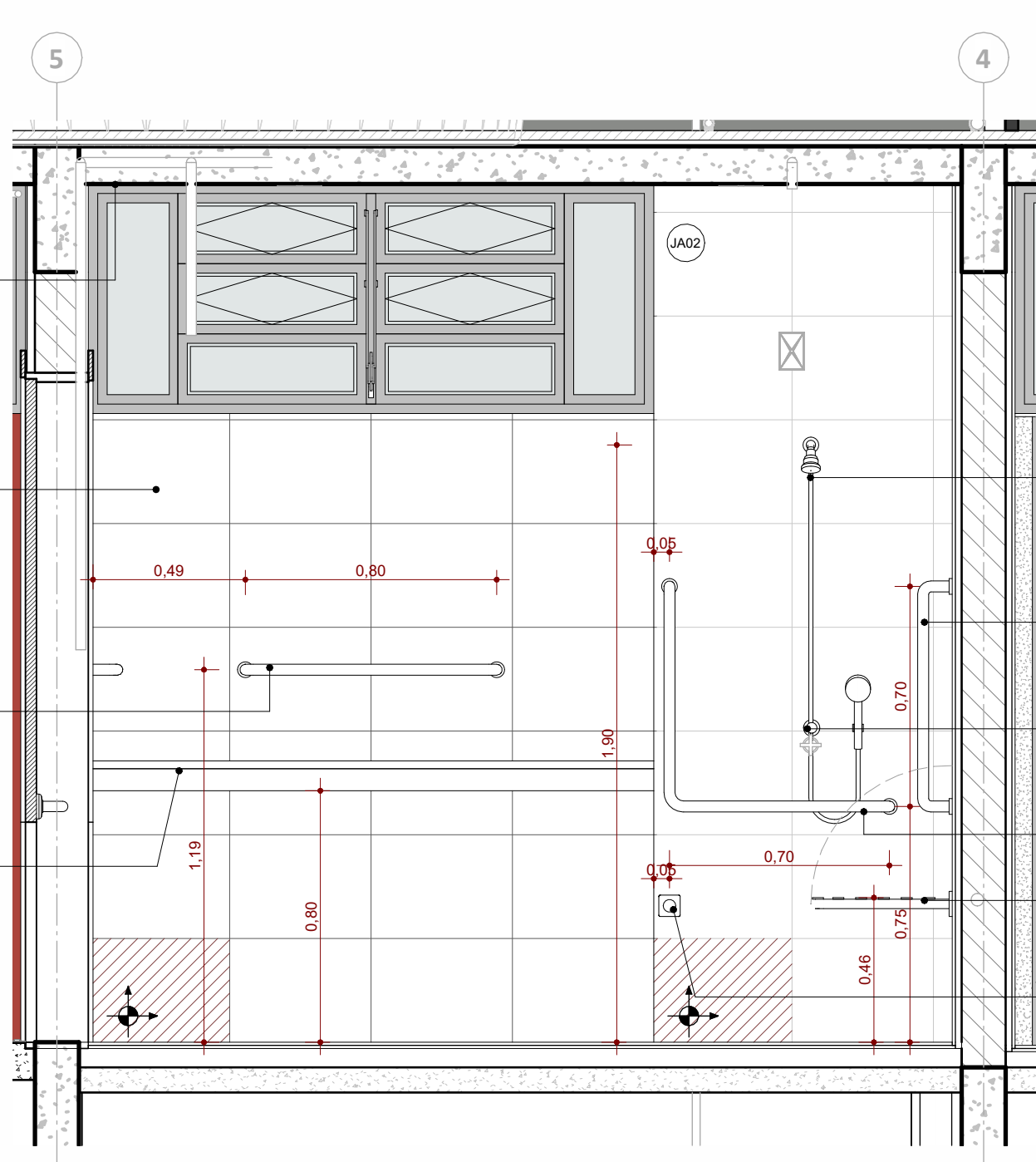
VISTA 07
