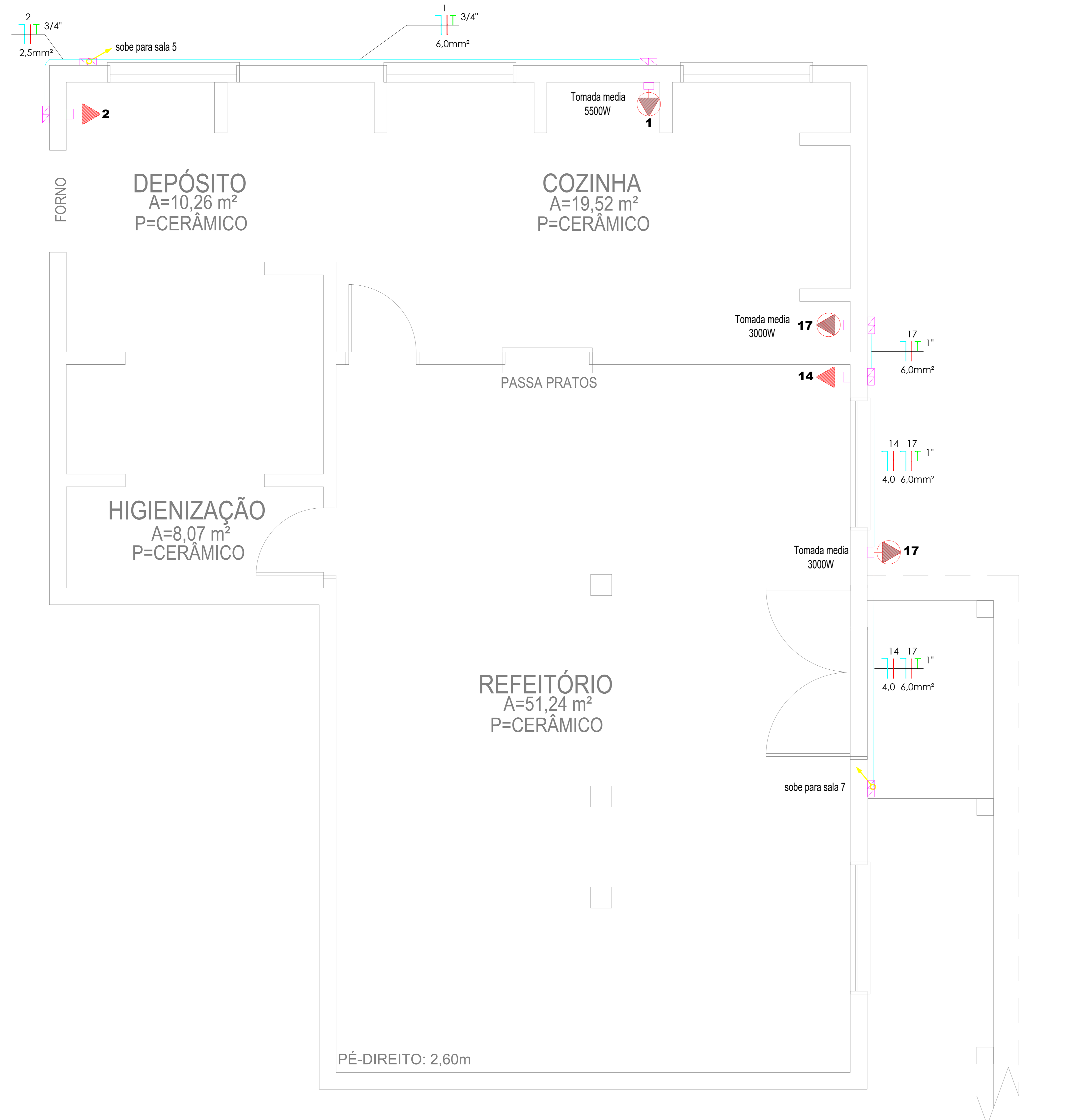
PLANTA BAIXA SUBSOLO ESCALA: 1/125 ÁREA TOTAL: 99,46 m 2
