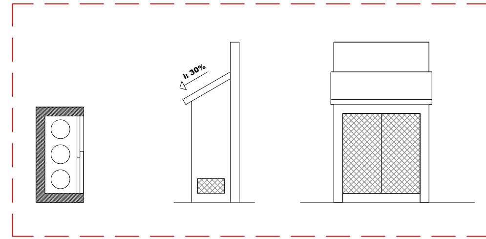
02 DETALHE 01 - CENTRAL DE GÁS Escala 1/50
