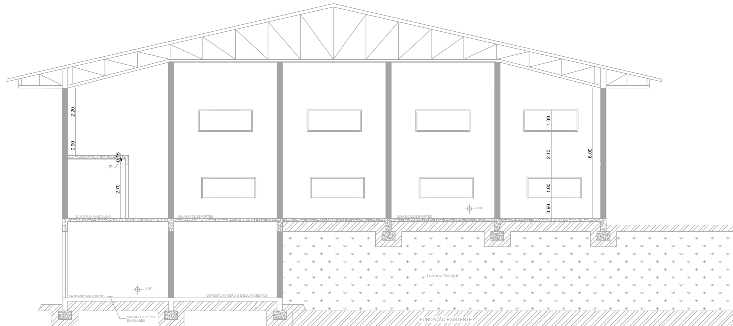
CORTE BB' ESCALA: 1/100
