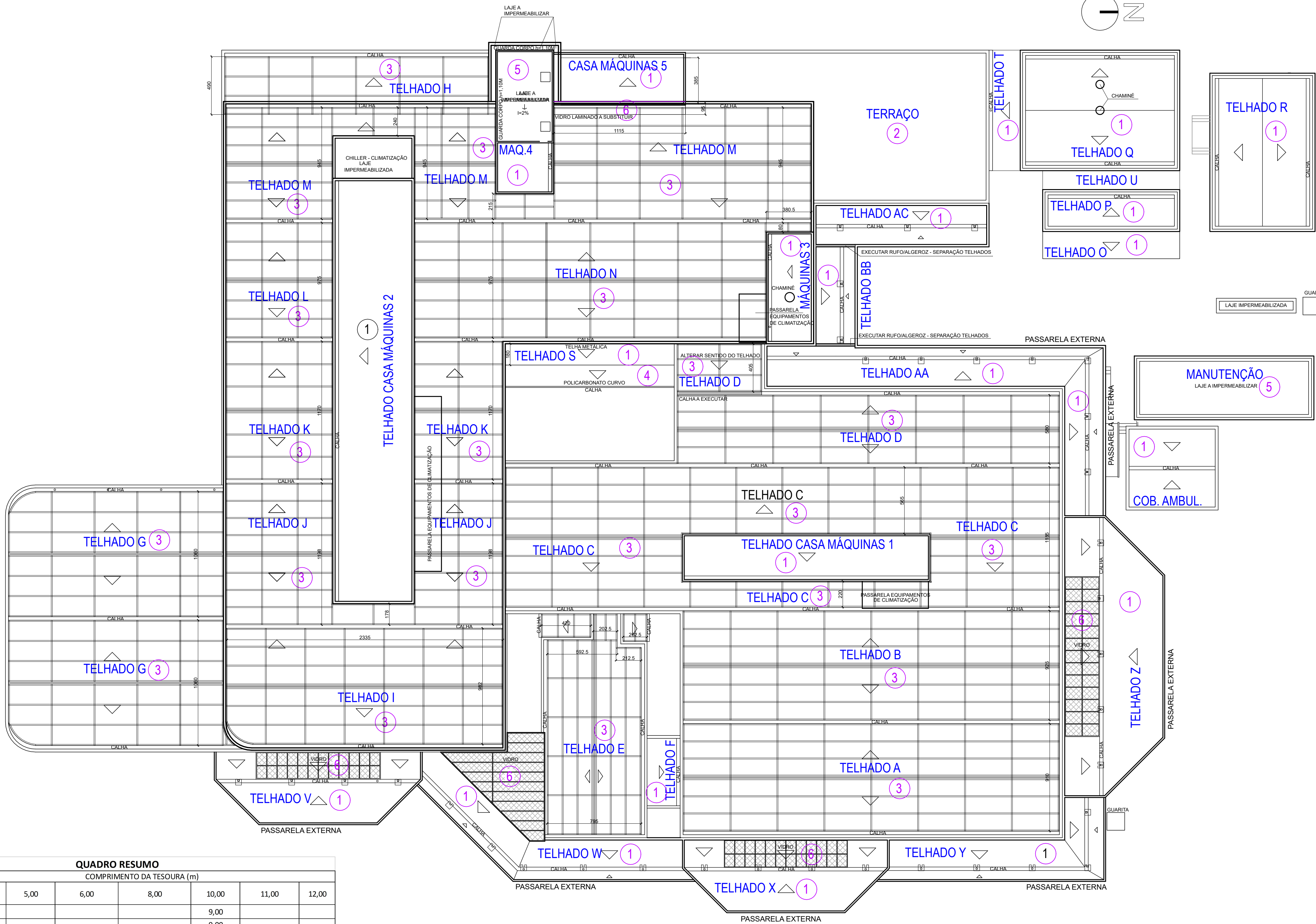
PLANTA DE COBERTURA INDICAÇÃO DE LOCALIZAÇÃO DAS TESOURAS E TERÇAS ESCALA: 1/200
