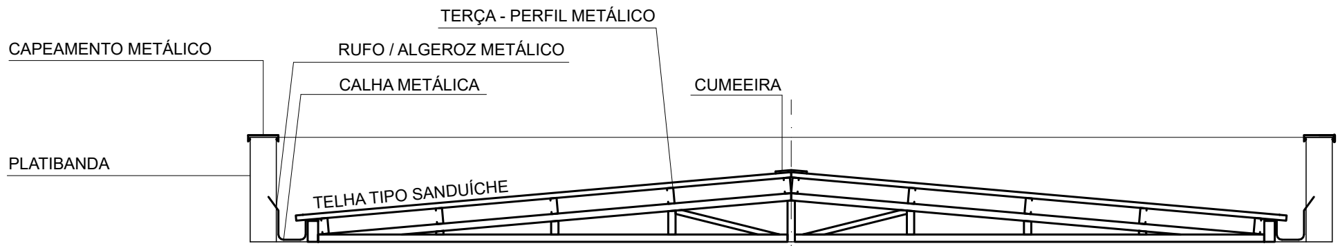
SEÇÃO TÍPICA DA COBERTURA - TESOURA, TERÇAS, CALHA, TELHA, ALGEROZ E RUFO SEM ESCALA
