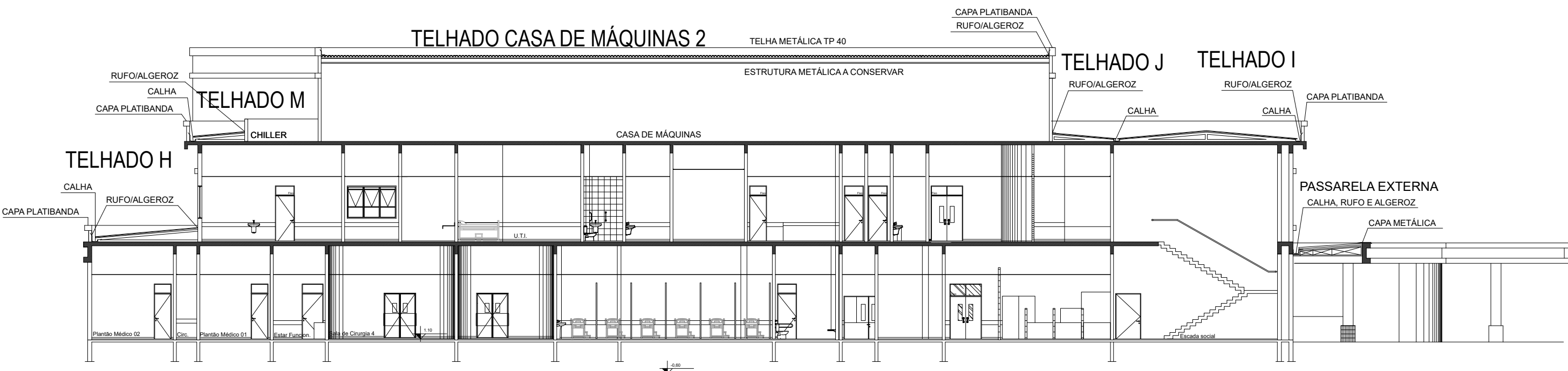
CORTE ESQUEMÁTICO D-D ESCALA: 1/100
