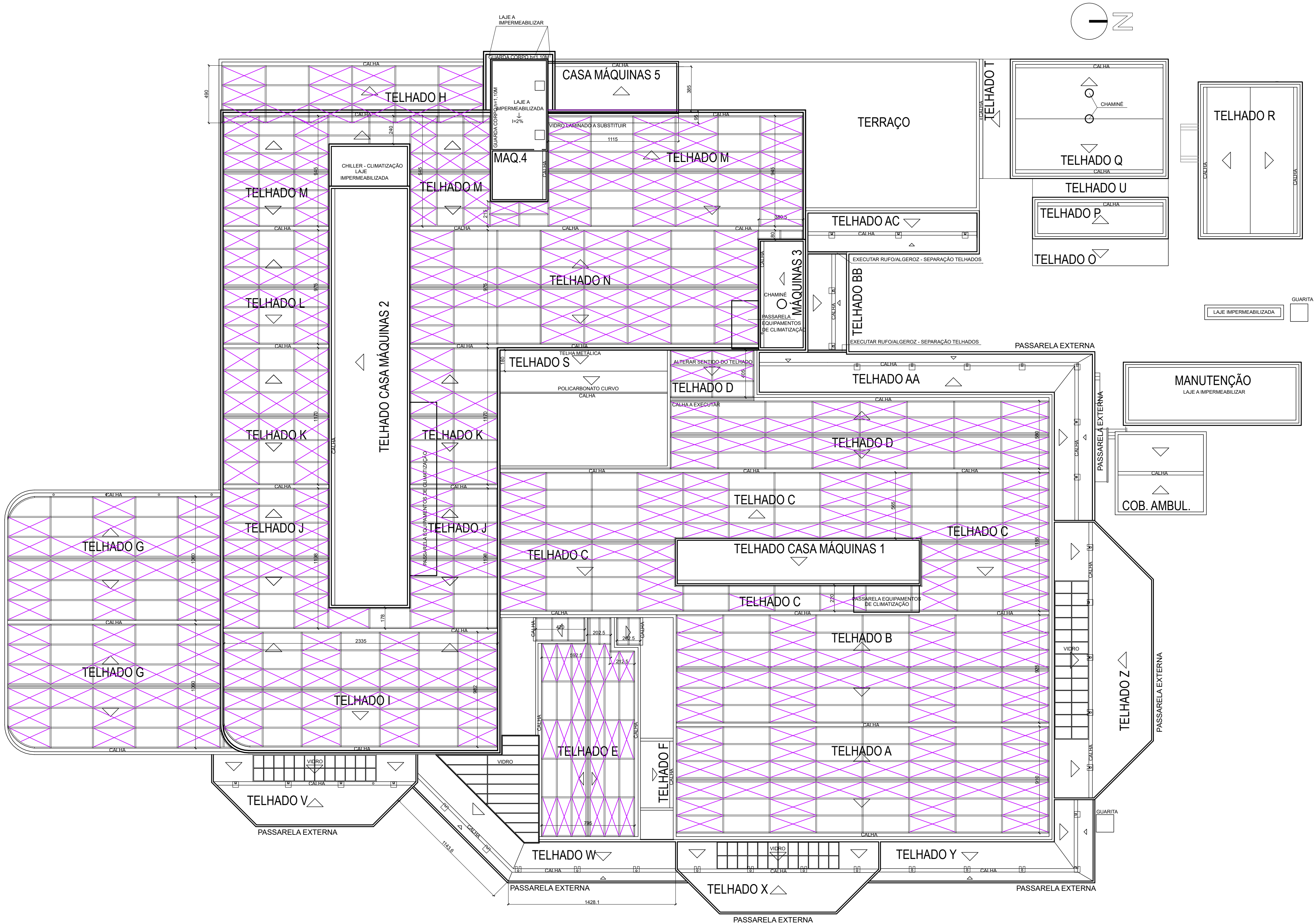
PLANTA DE COBERTURA CONTRAVENTAMENTO HORIZONTAL ESCALA: 1/200
