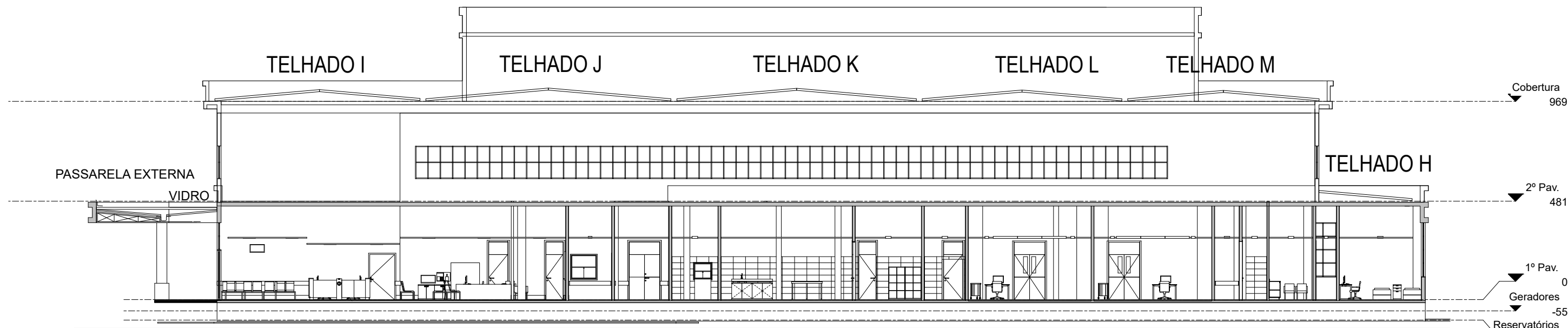
CORTE ESQUEMÁTICO B-B ESCALA: 1/100
