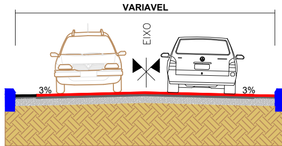
SEÇÃO TIPO DE PAVIMENTAÇÃO SEM ESCALA
