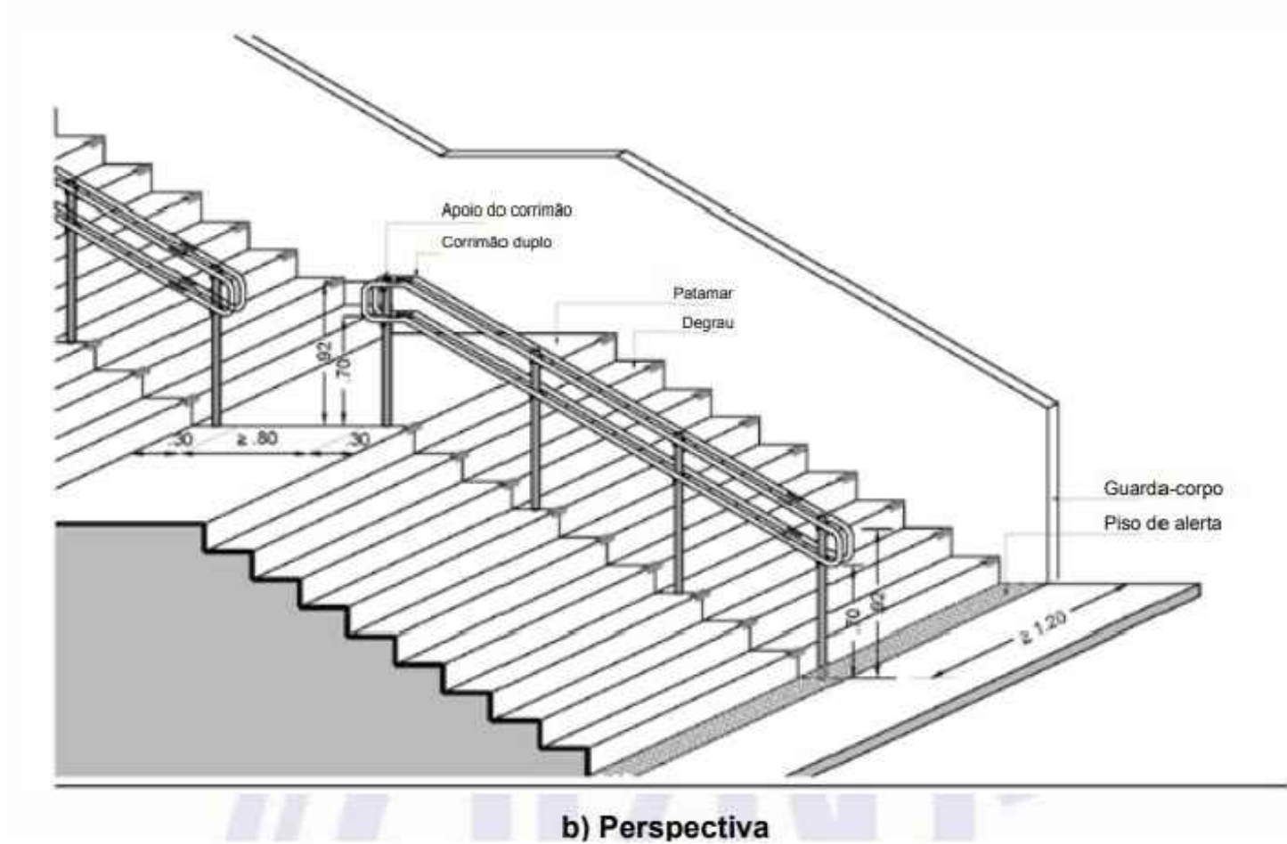
Detalhamento Guarda-Corpos - Padrão NBR 9050
