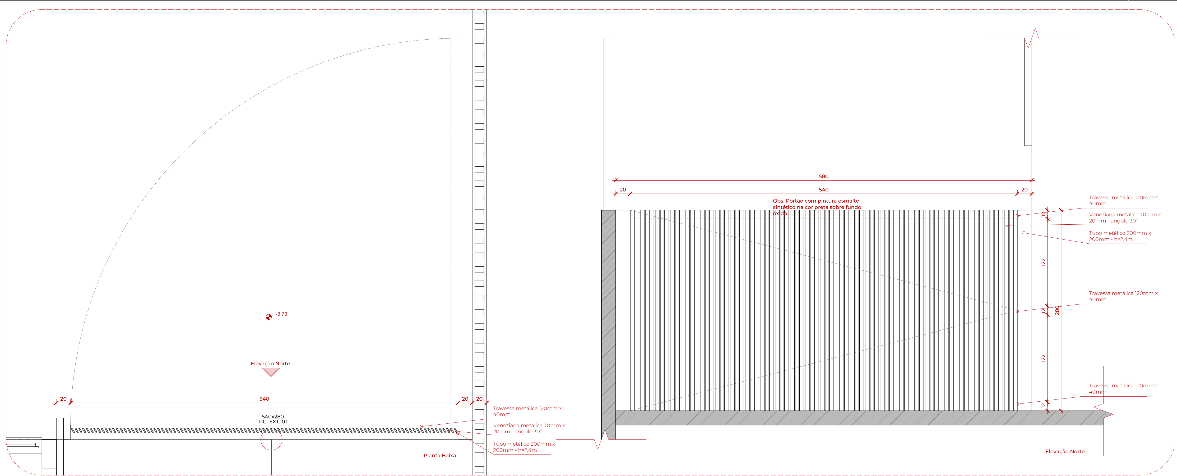
Detalhamento Específico 04 - Portão Externo
