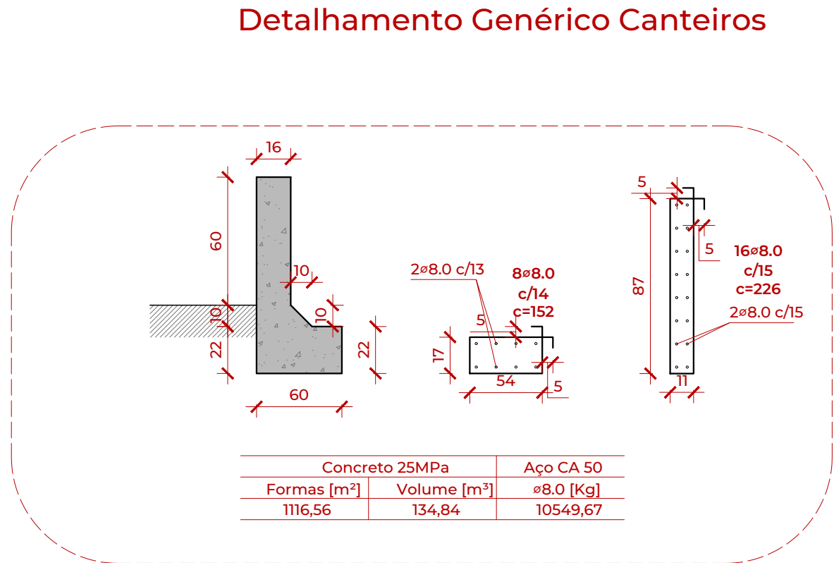
Detalhamento Genérico Parede Canteiros
