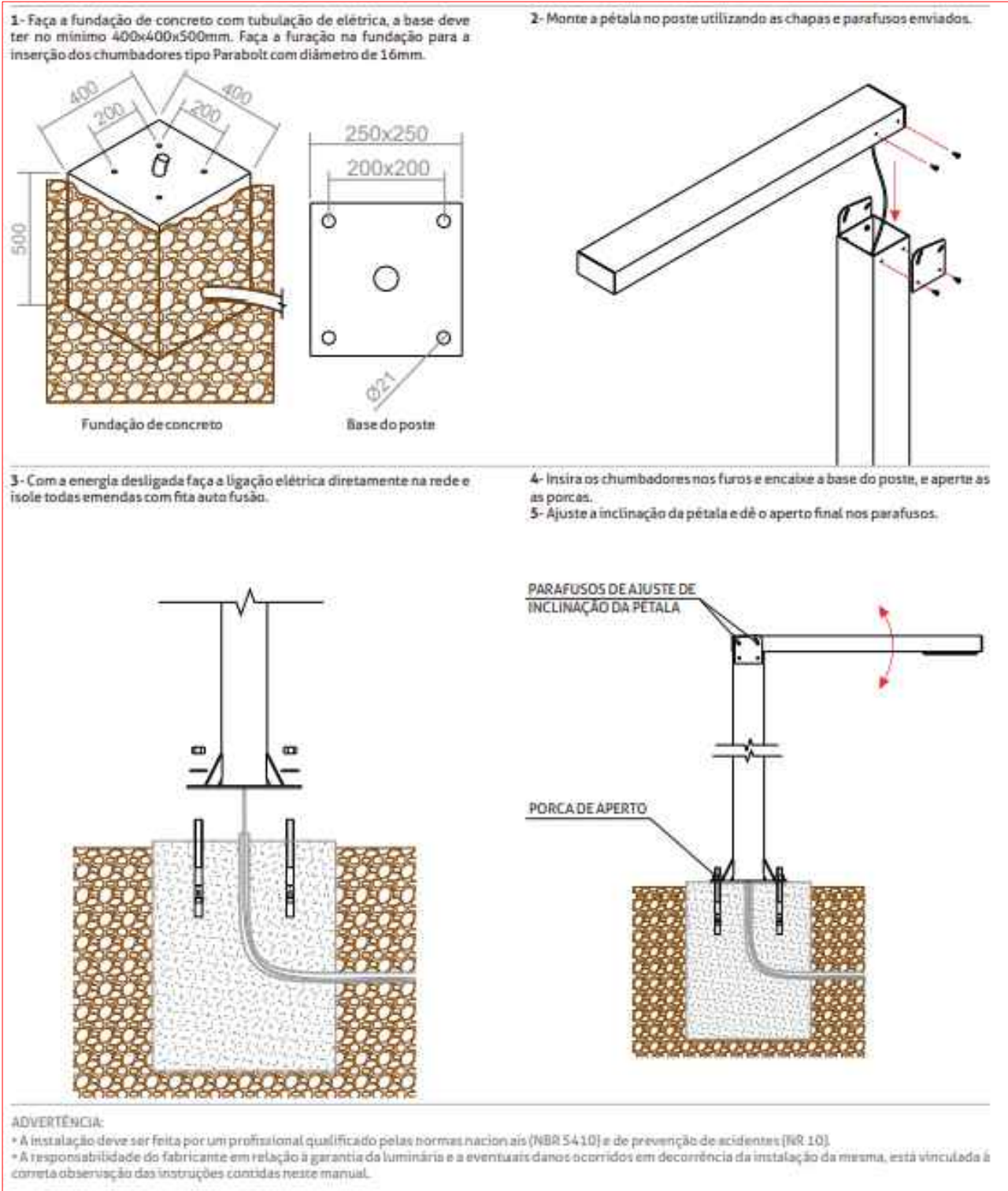
Detalhe Instalação Poste de Iluminação Simples
