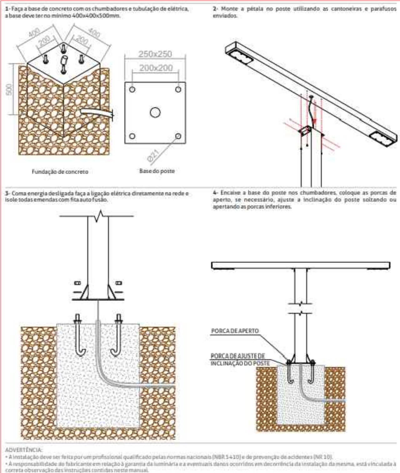
Detalhe Instalação Poste de Iluminação Duplo
