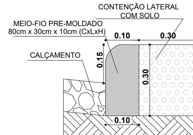
DETALHAMENTO DO MEIO-FIO ESC:S/E
