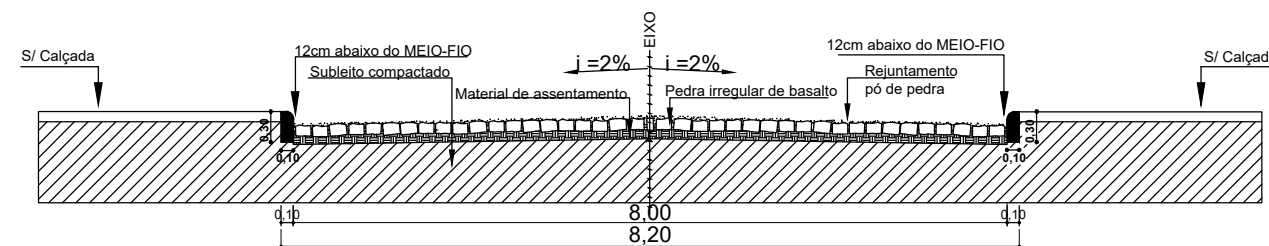
PERFIL TRANSVERSAL ESC:S/E
