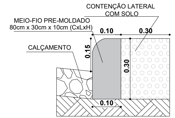
DETALHAMENTO DO MEIO-FIO ESC:S/E
