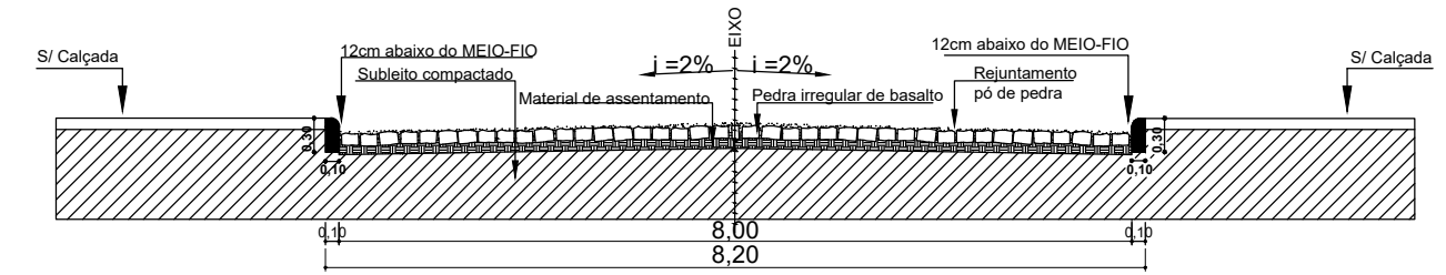
PERFIL TRANSVERSAL ESC:S/E
