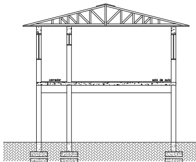
CORTE B - B
