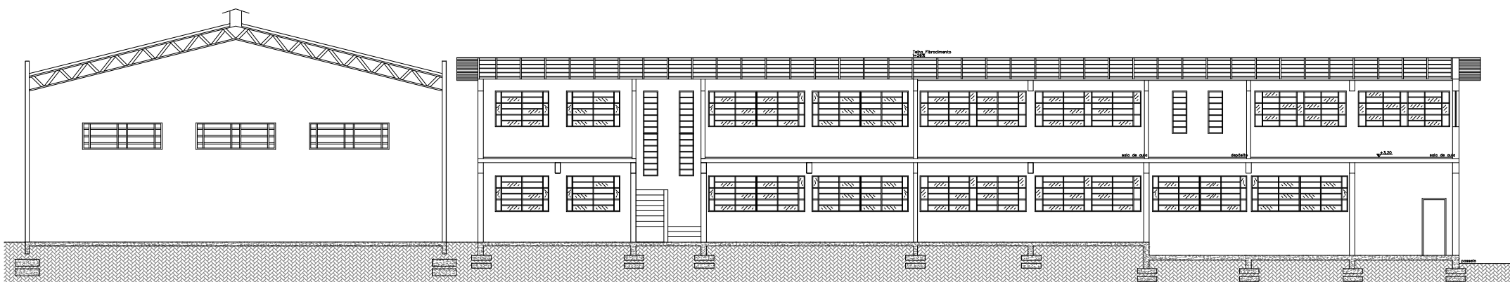
CORTE A - A
