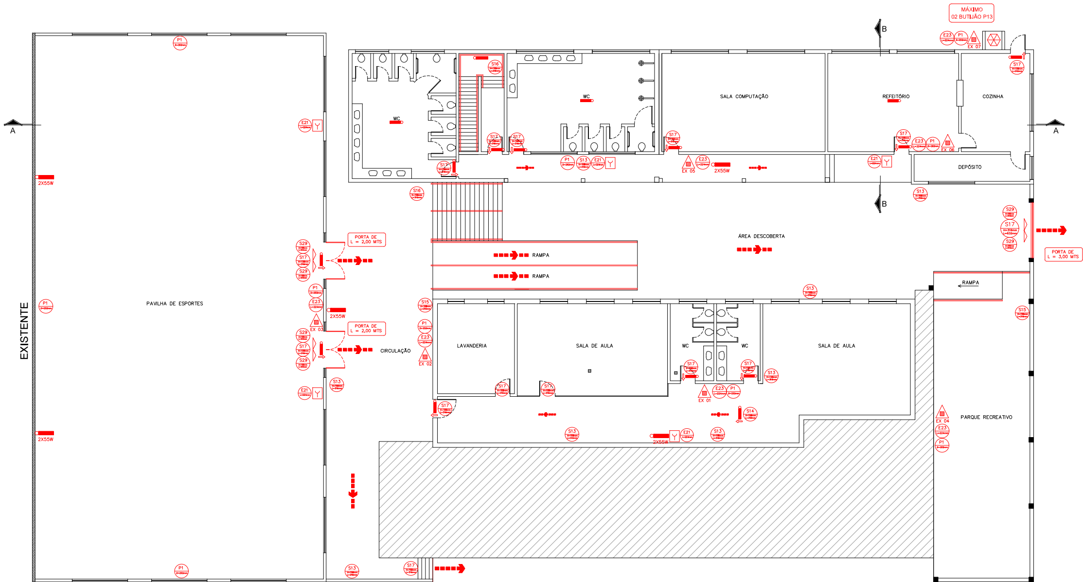
PLANTA BAIXA 1º ANDAR
