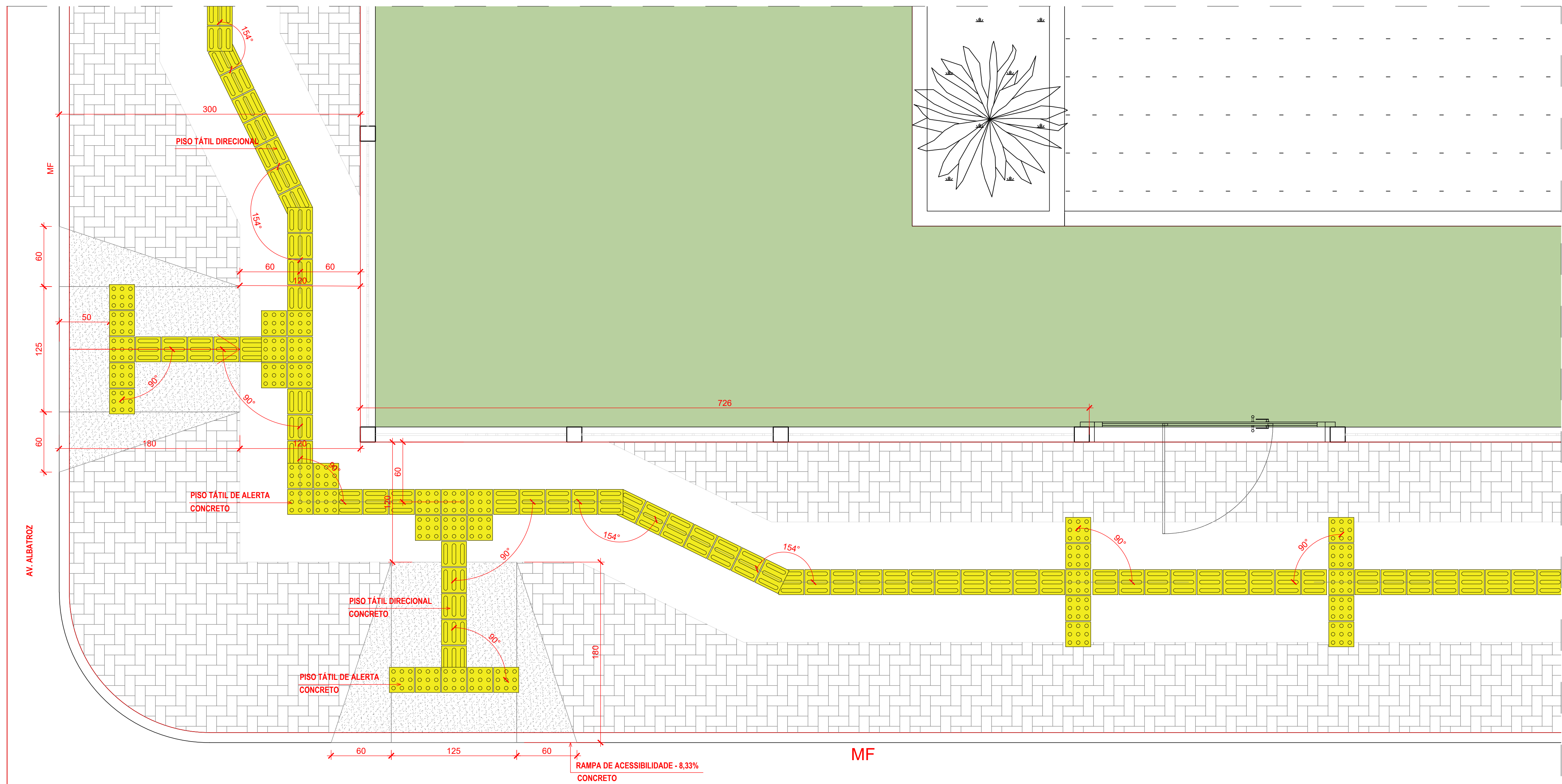
DETALHE 02 - CALÇADA AV. ALBATROZ X RUA LUIZINHO E ACESSO POSTERIOR DE PEDESTRES ESC.: 1/25
