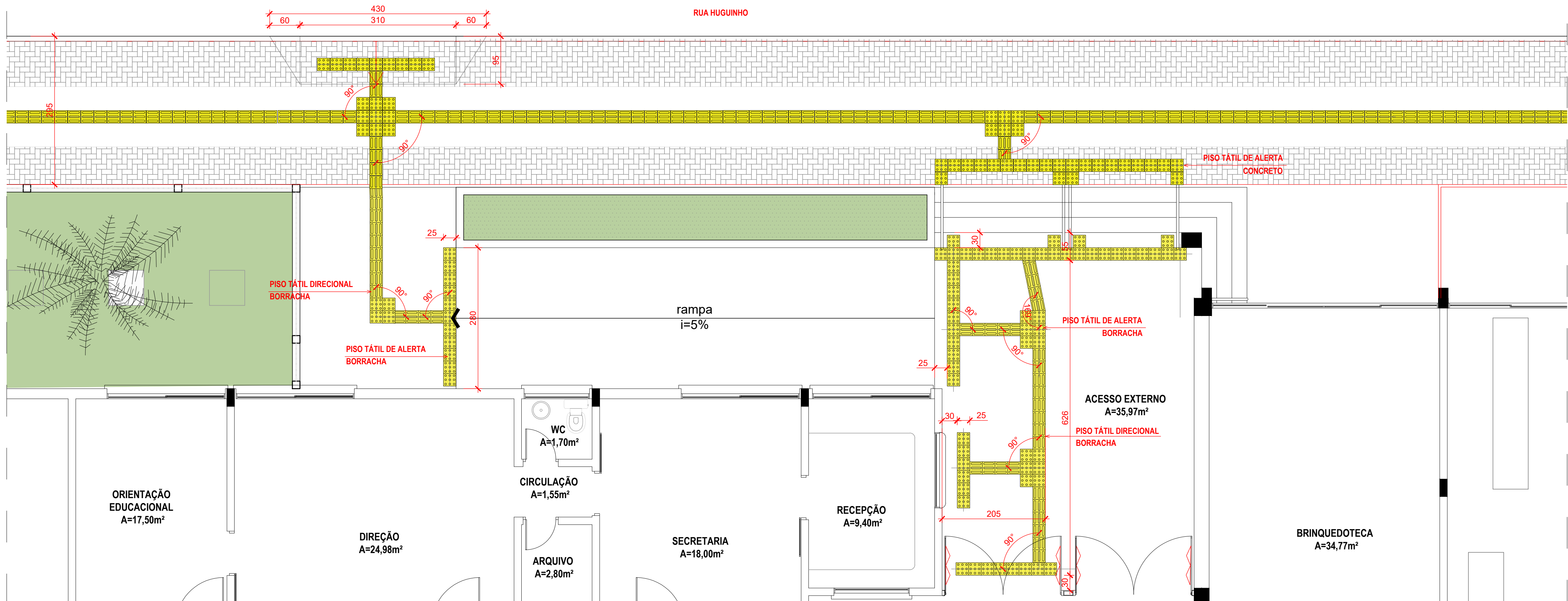
DETALHE 01 - ACESSO FRONTAL RUA HUGUINHO ESC.: 1/50
