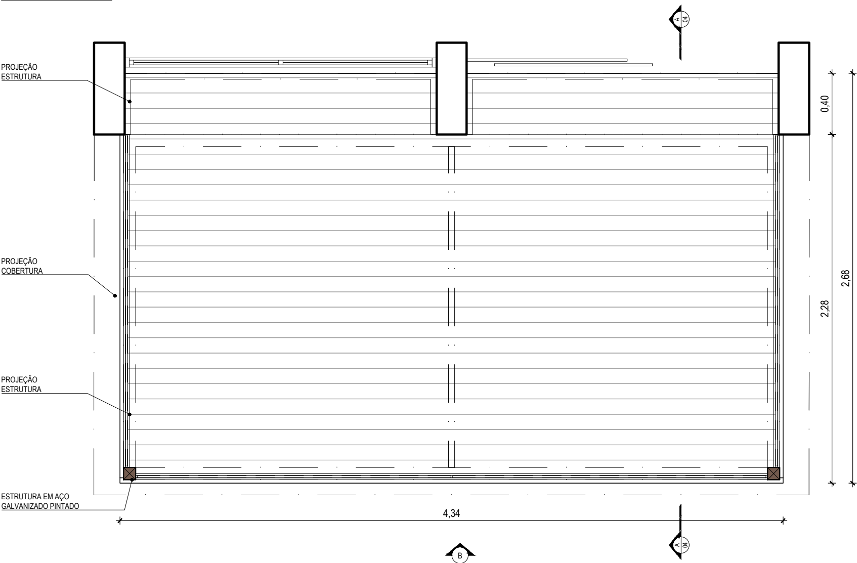
01 PLANTA BAIXA - DECK NORTE - RESTAURANTE B ESC: 1/25
