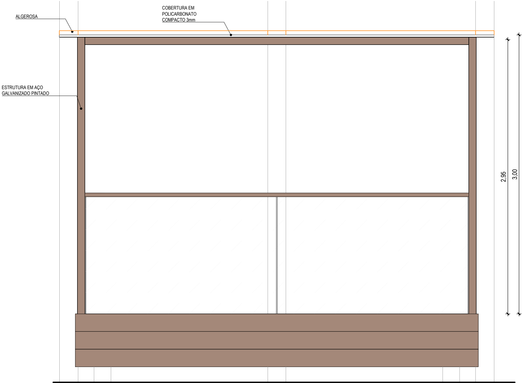
03 VISTA B - DECK NORTE - RESTAURANTE B ESC: 1/25
