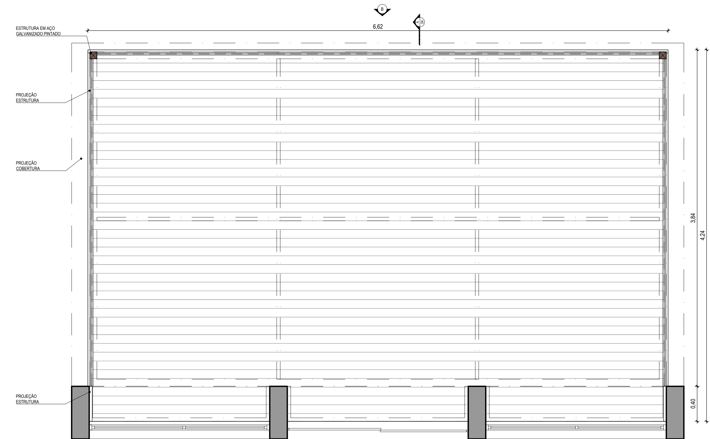
01 PLANTA BAIXA - DECK SUL - RESTAURANTE A ESC: 1/25
