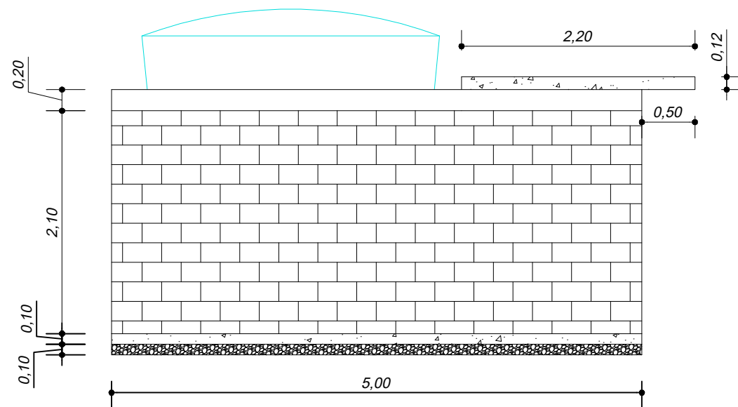
FACHADA 1:50
