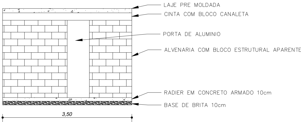
FACHADA 1:50
