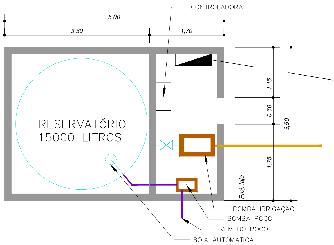
PLANTA BAIXA 1:50
