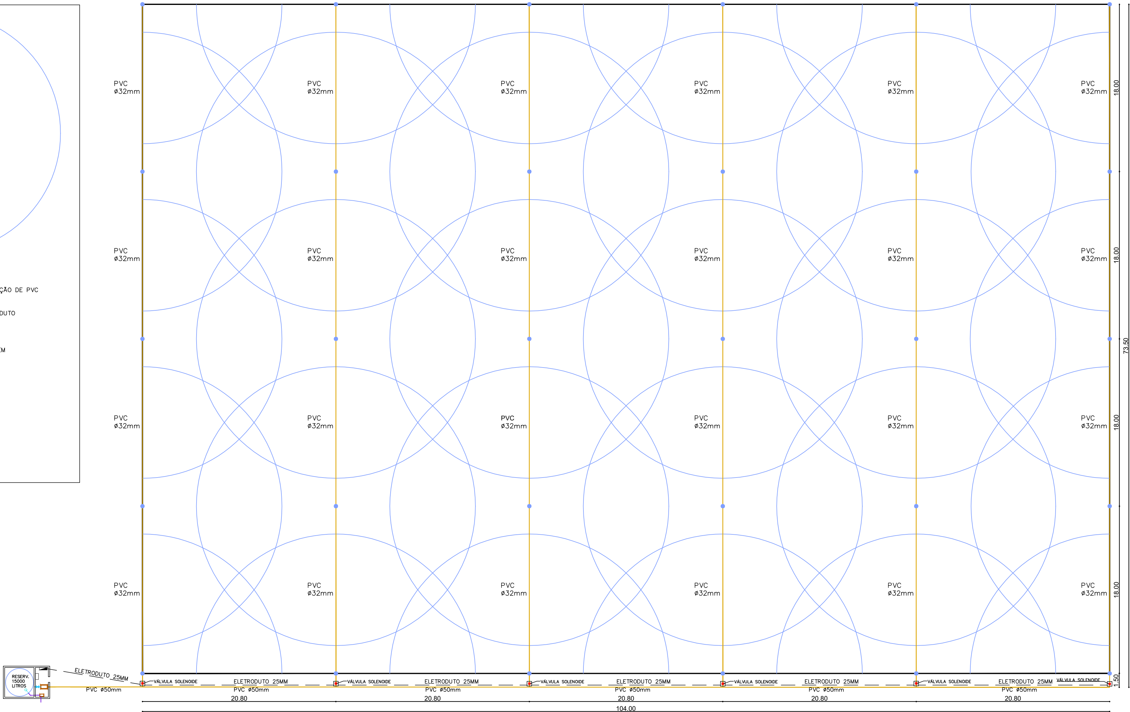
IRRIGAÇÃO CAMPO DE FUTEBOL 1:250
