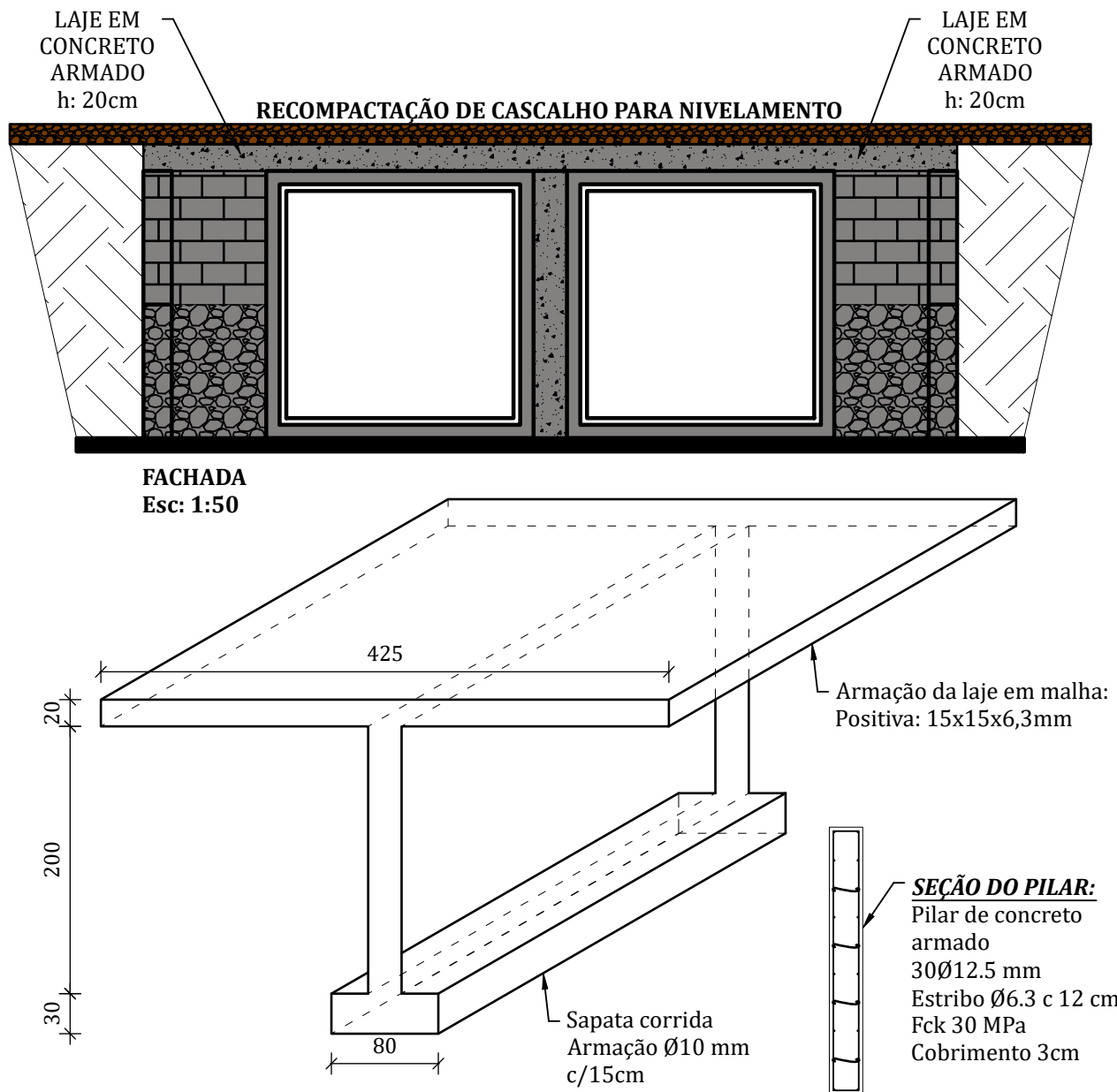
PERSPECTIVA DA ESTRUTURA EM CONCRETO ARMADO Esc: 1:50
