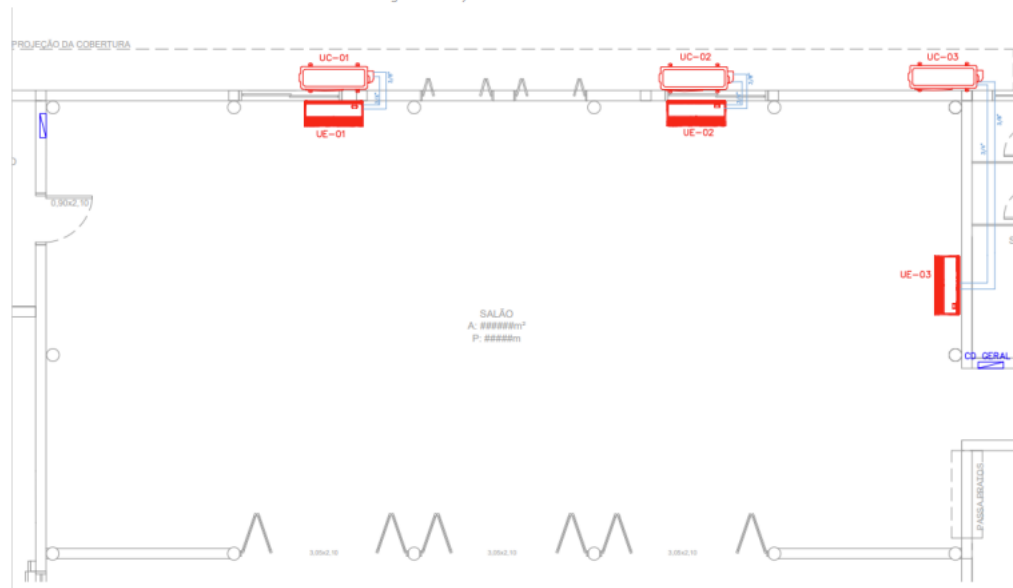
Figura 2 – Layout Unidades Climatizadoras
