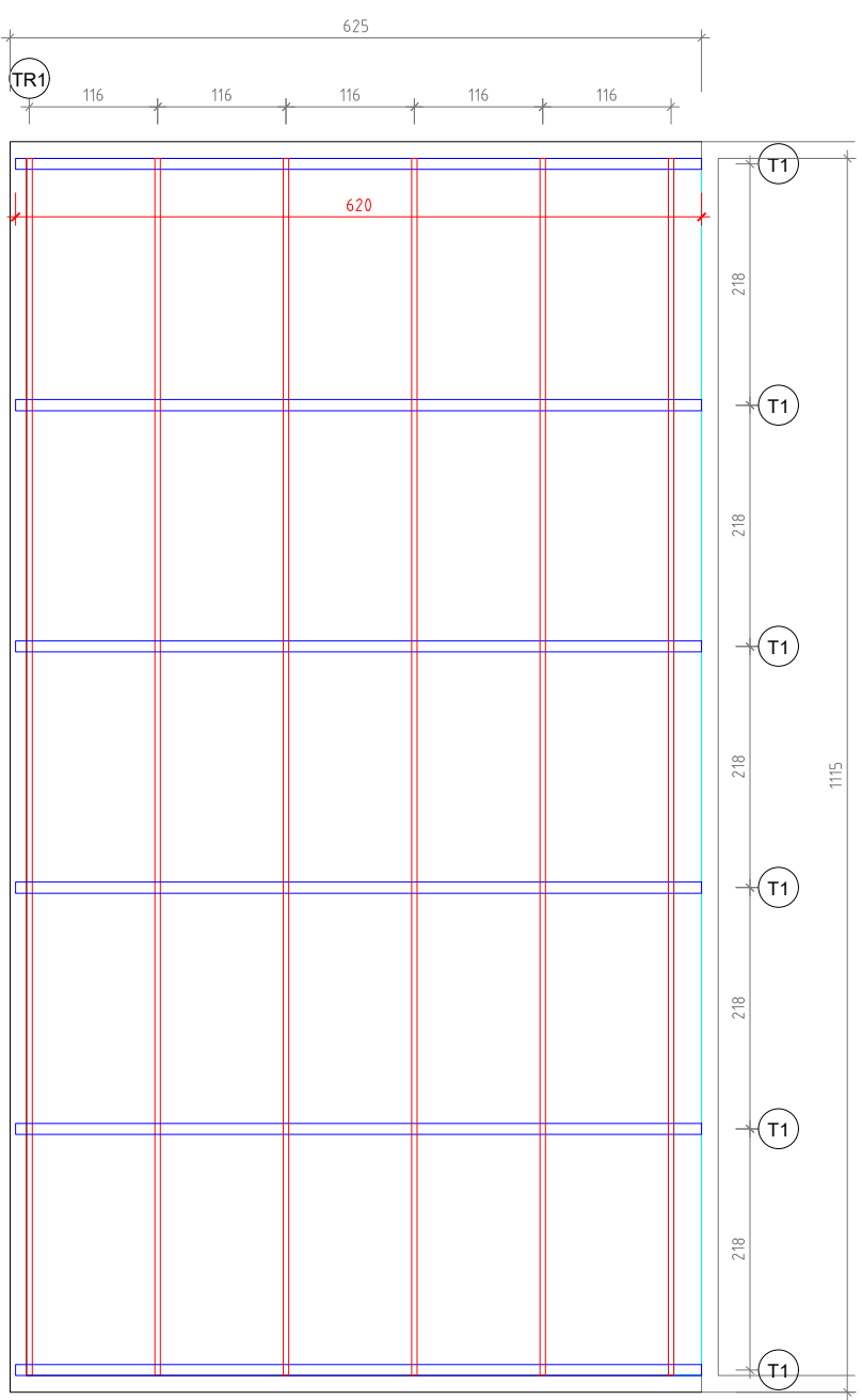
Projeto Estrutural COBERTURA GABINETE A=49,68m² Esc: 1/50
