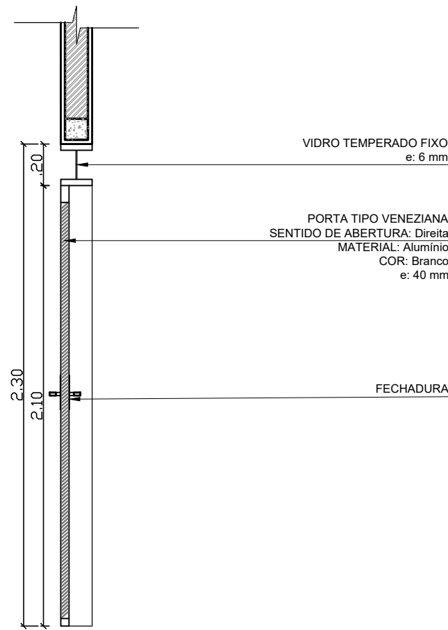
CORTE esc 1:25
