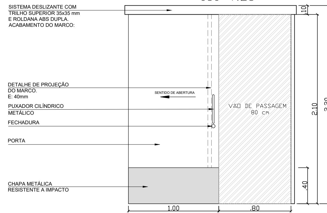
DETALHAMENTO P1 (aberta) esc 1:25
