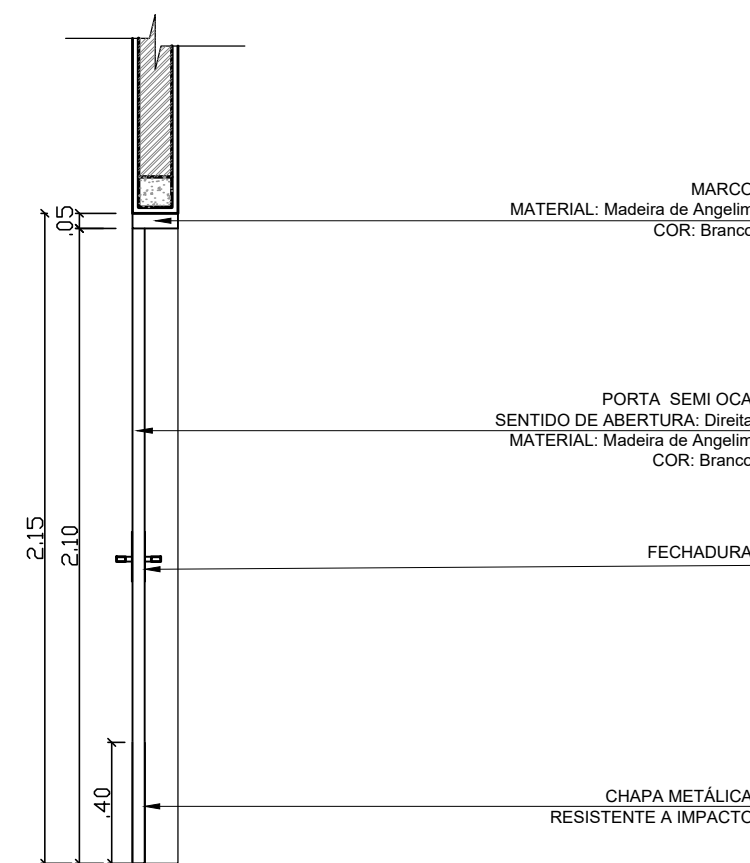
CORTE esc 1:25
