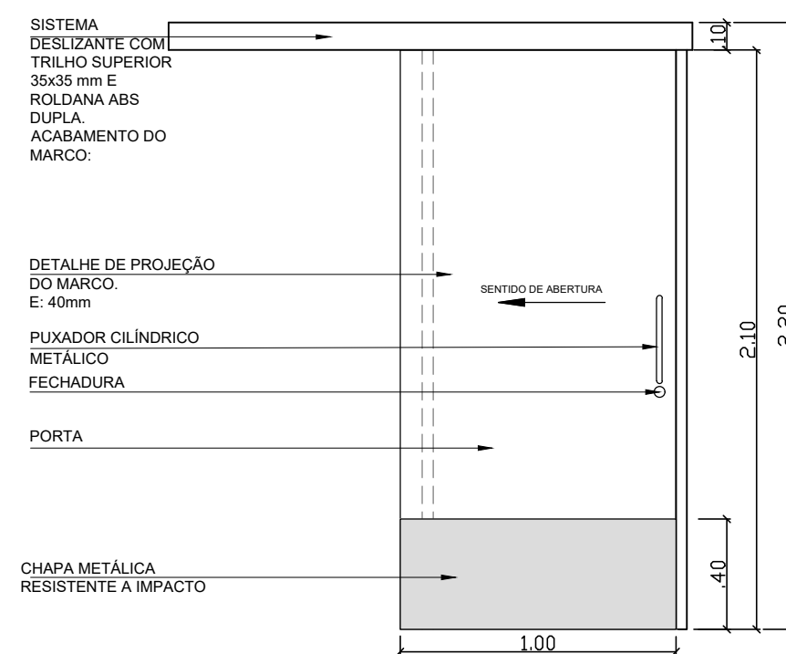
DETALHAMENTO P1 (fechada) esc 1:25
