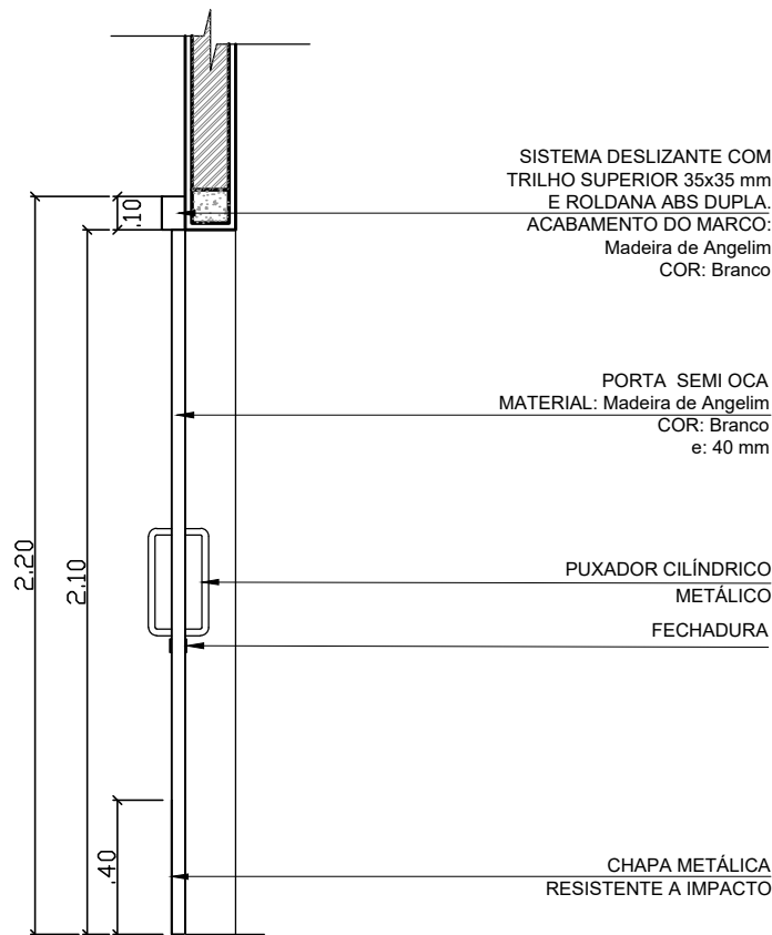
CORTE esc 1:25
