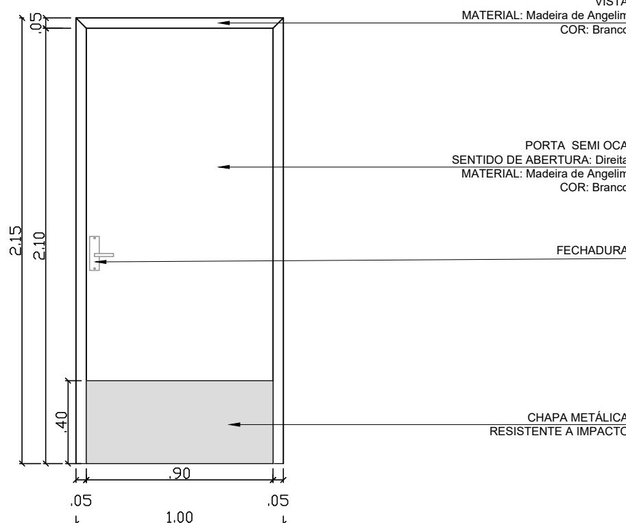
DETALHAMENTO P2 esc 1:25
