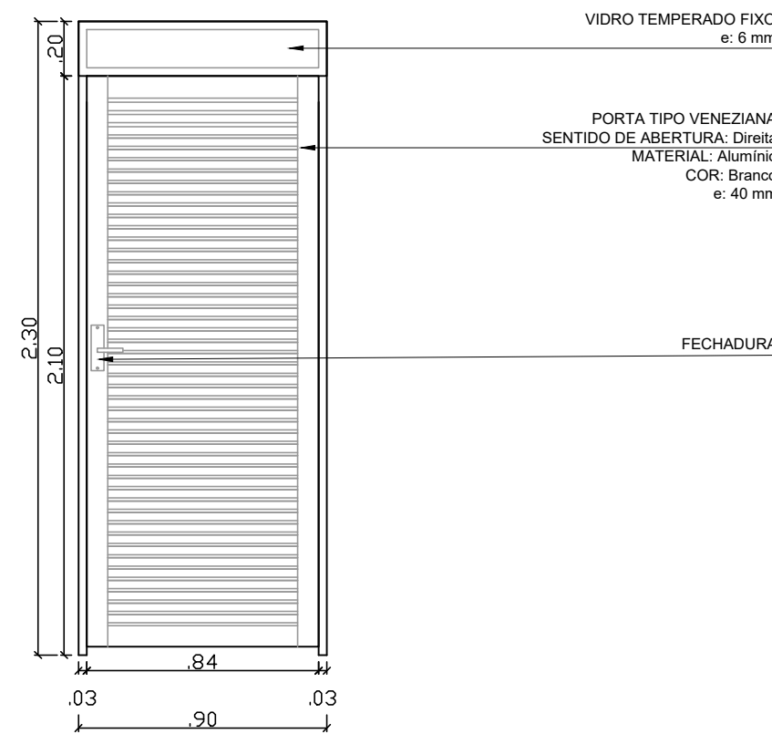
DETALHAMENTO P1 esc 1:25
