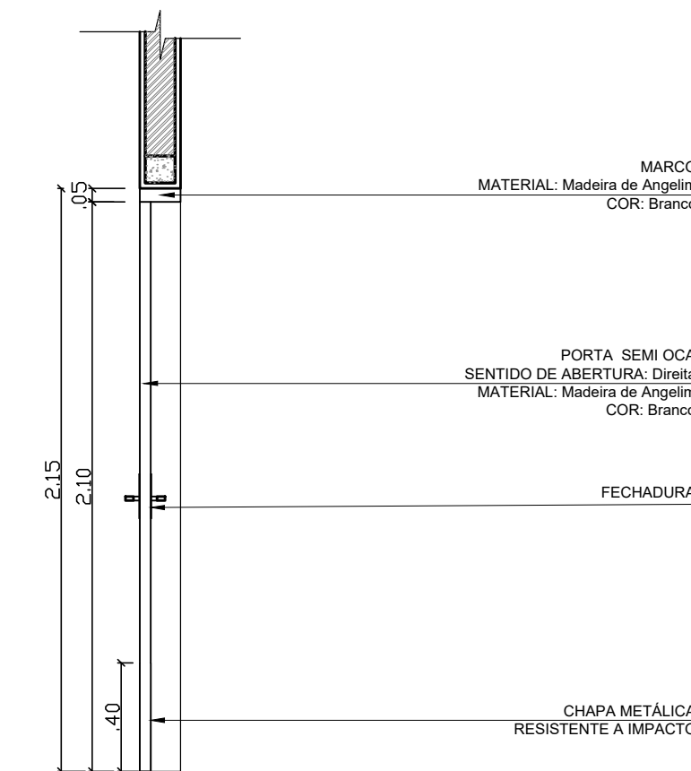
CORTE esc 1:25
