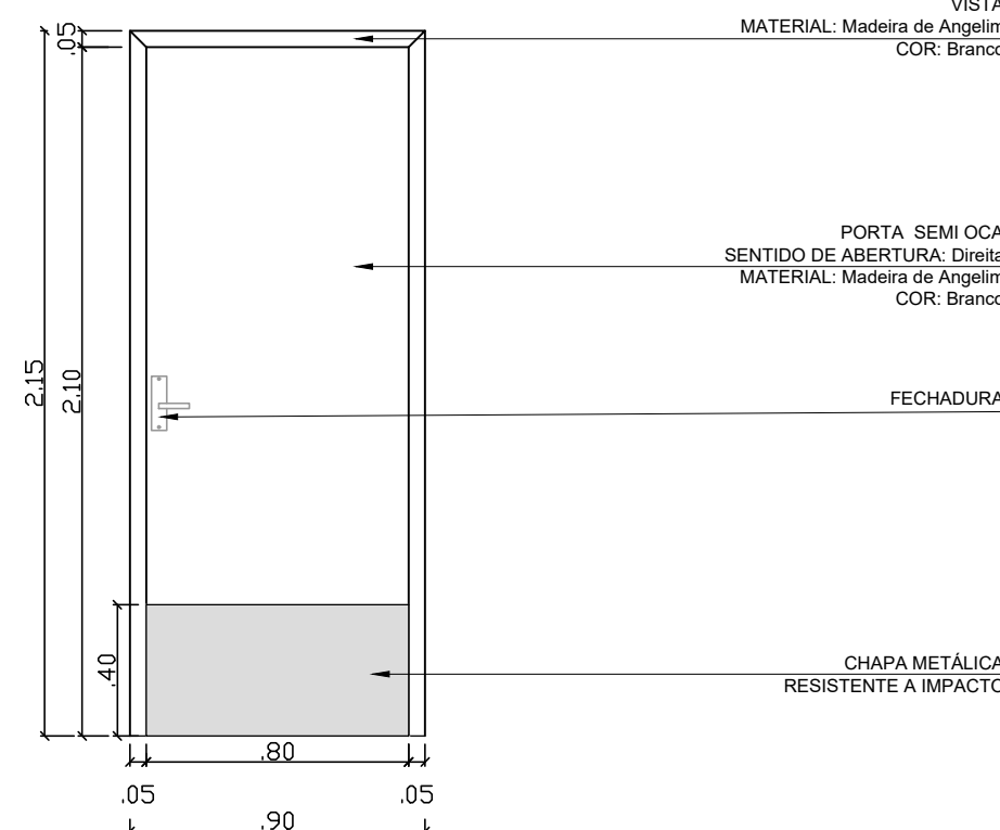
DETALHAMENTO P3 esc 1:25
