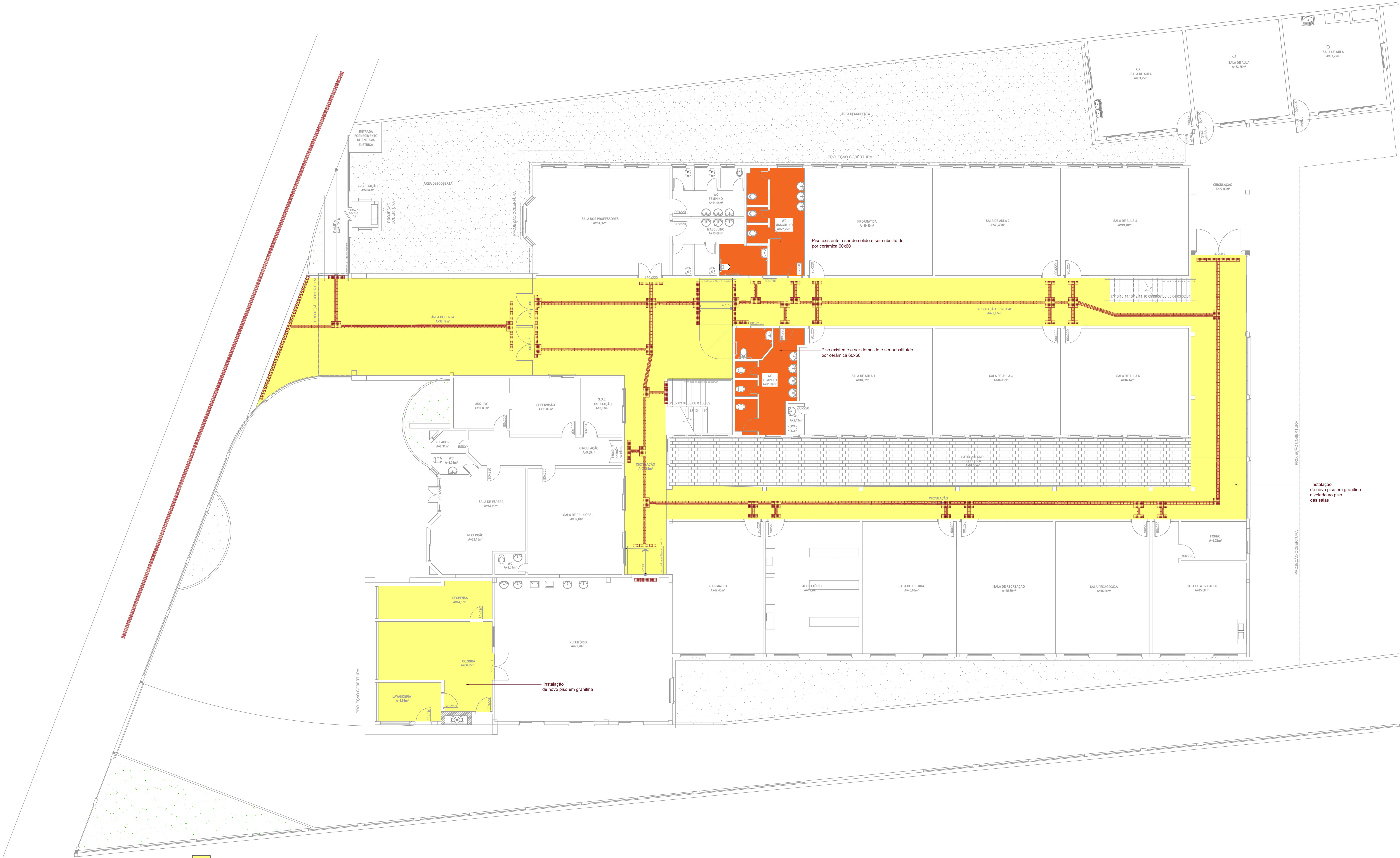
PLANTA BAIXA PAVIMENTO TERREO ESCOLA Esc.:1/100
