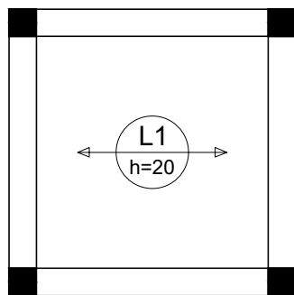
VIGOTA PROTENDIDA COM BLOCO CERÂMICO ESCALA 1:50
