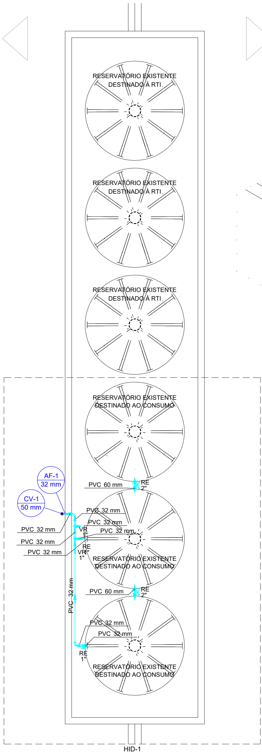
PLANTA BAIXA - CAIXAS D'ÁGUA Escala 1:50
