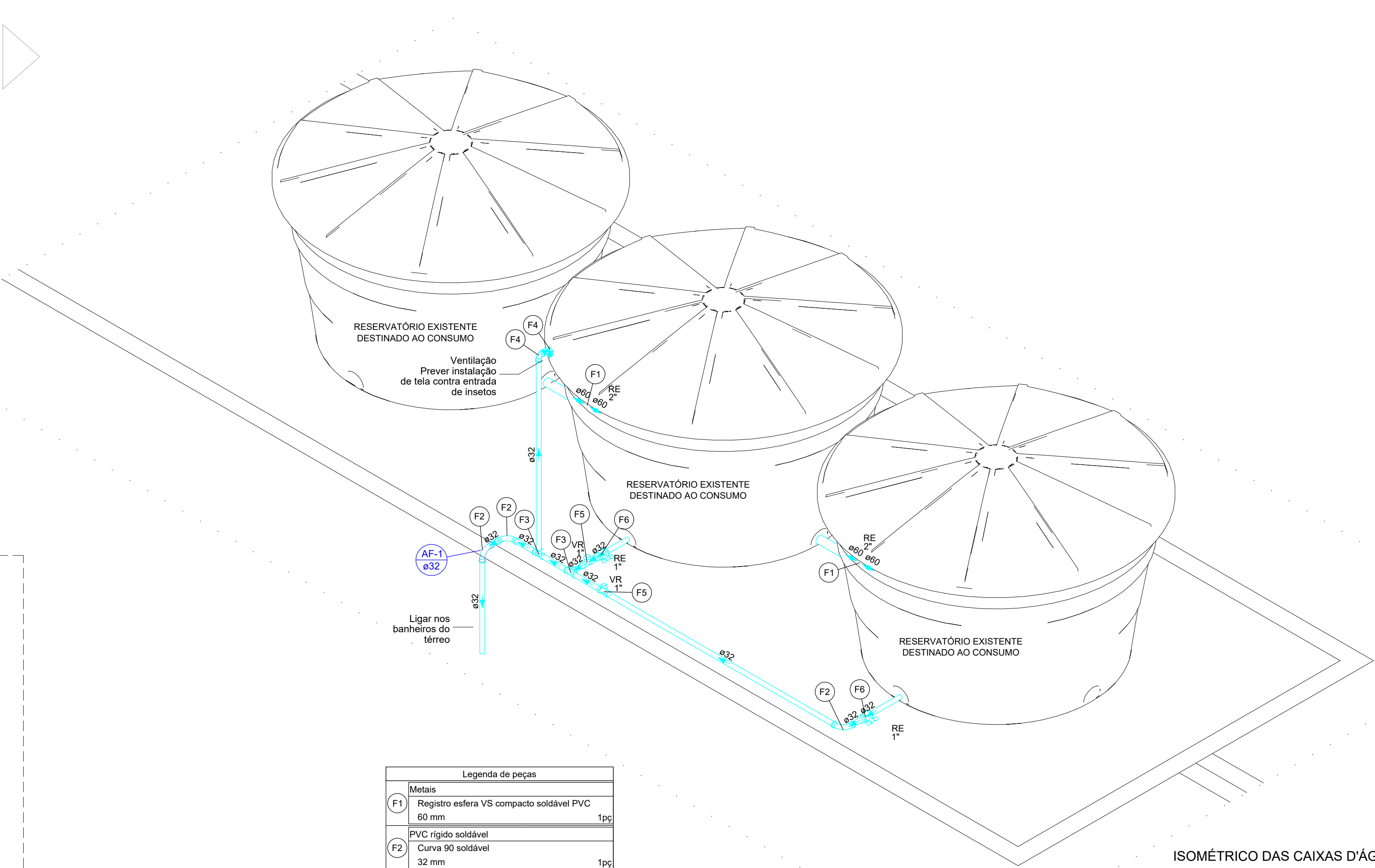
ISOMÉTRICO DAS CAIXAS D'ÁGUA Escala 1:25
