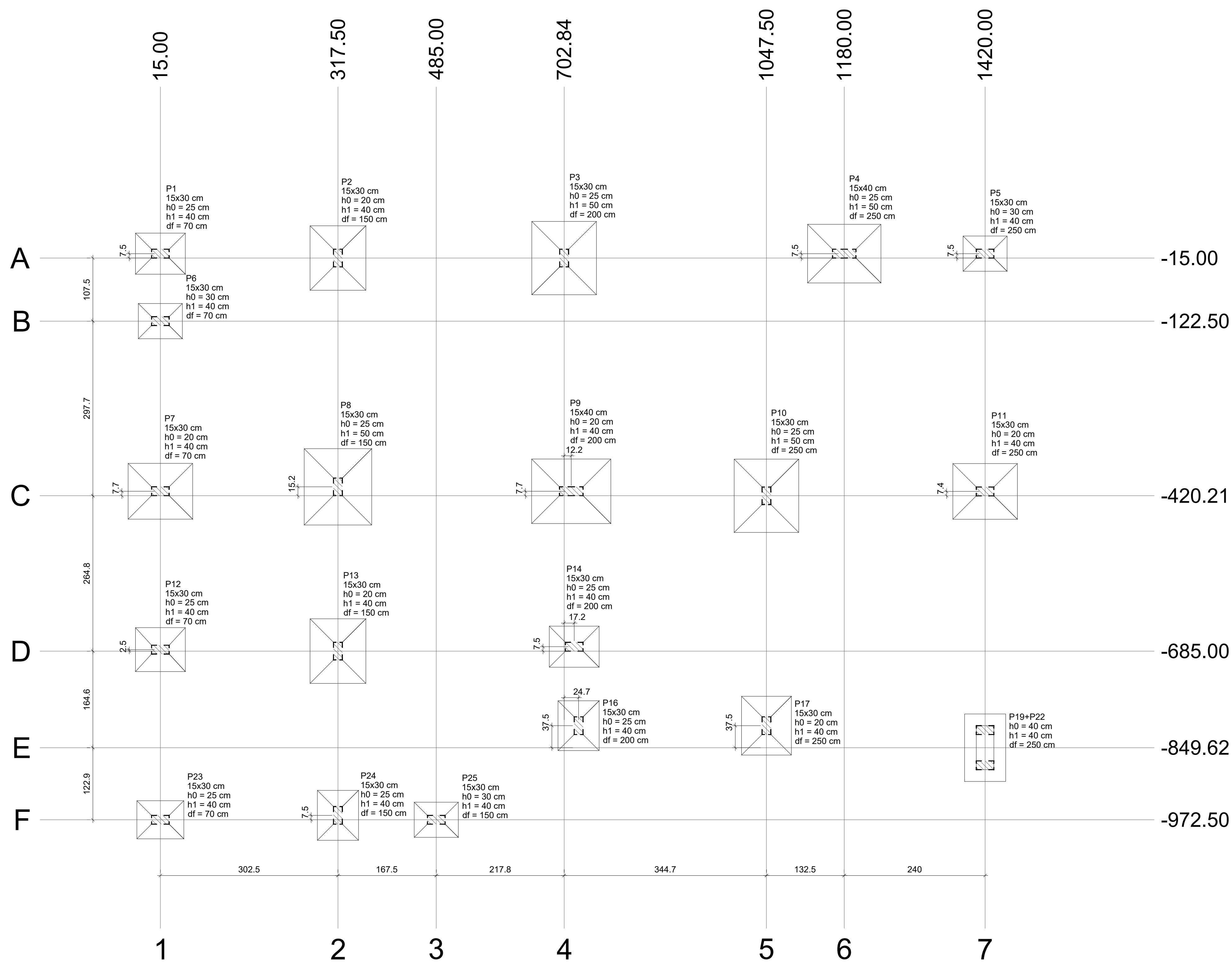
Planta de locação escala 1:50
