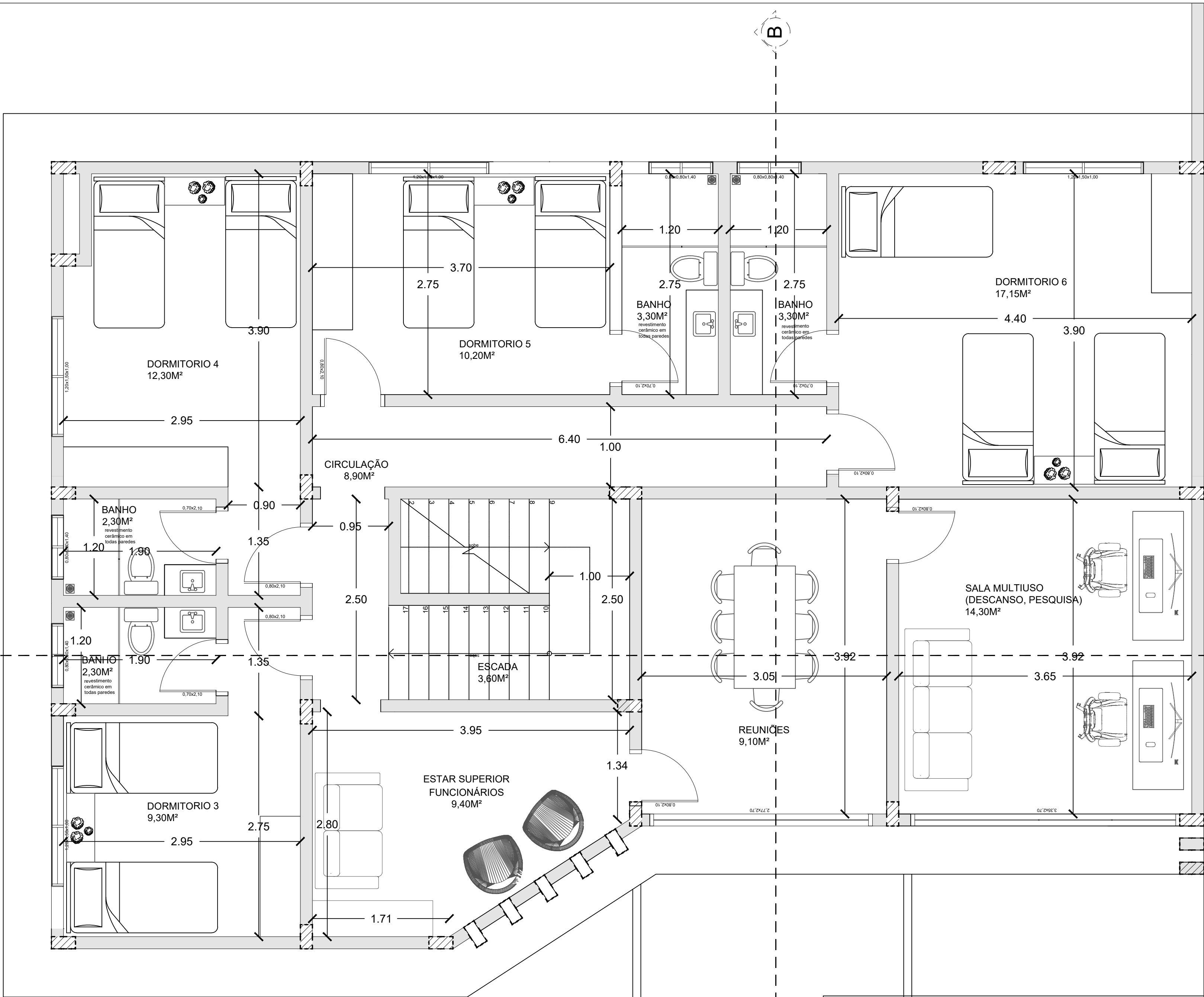
PLANTA BAIXA PAV. SUPERIOR ESC 1/35
