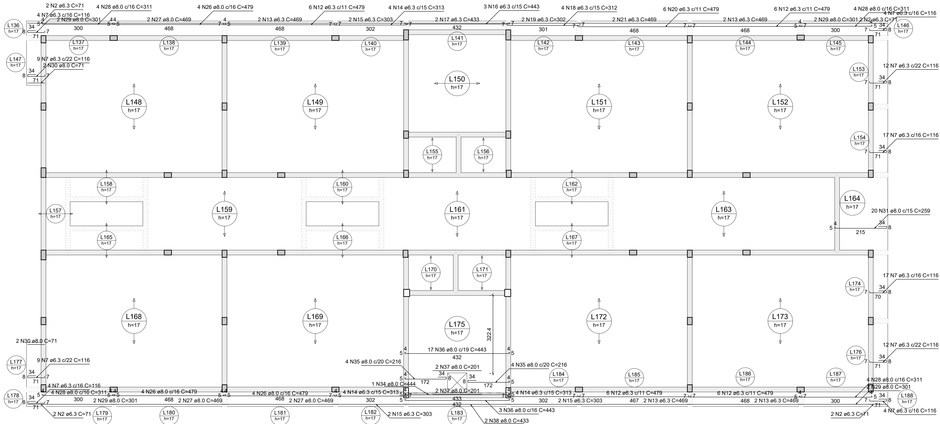
Armação positiva das lajes do pavimento Cobertura - blocos de salas (Eixo X)
