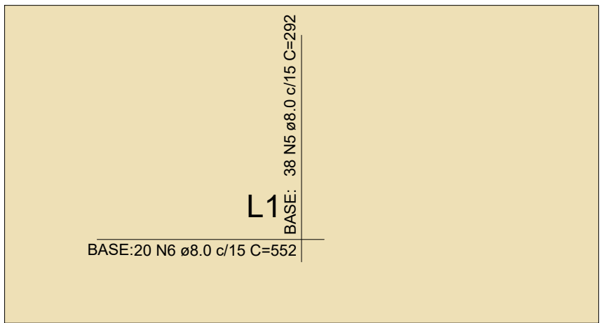
Armação superior do radier
