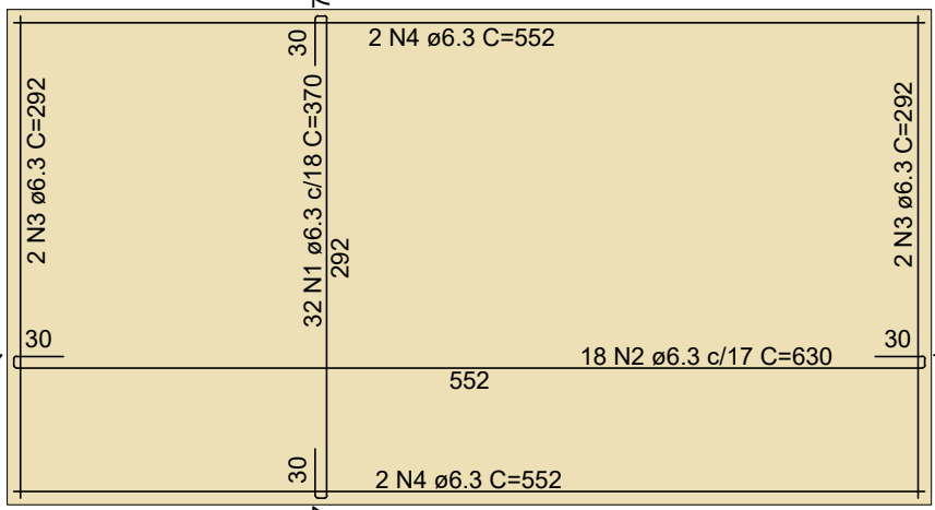
Armação inferior do radier
