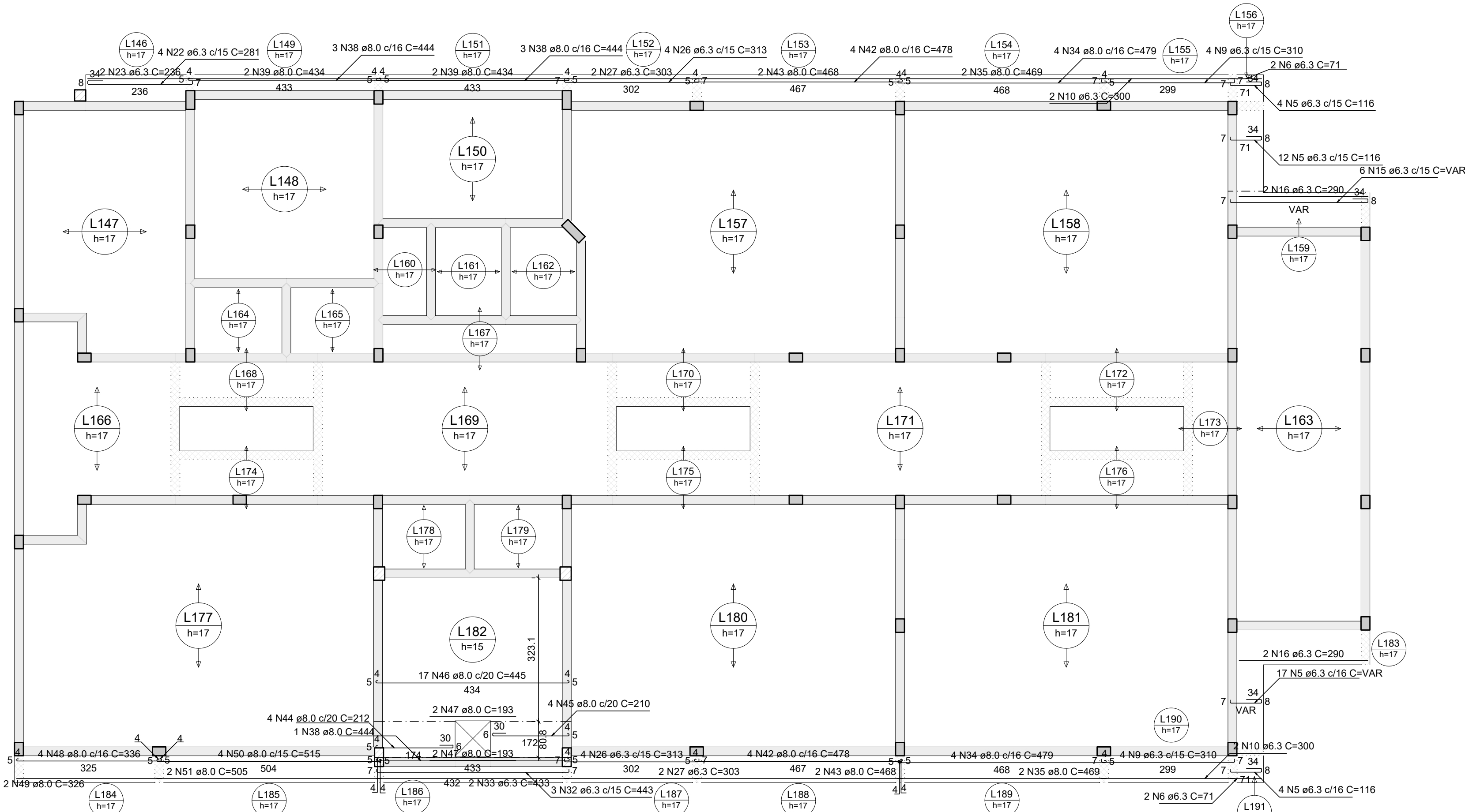
Armação positiva das lajes do pavimento Cobertura - blocos de salas (Eixo X)
