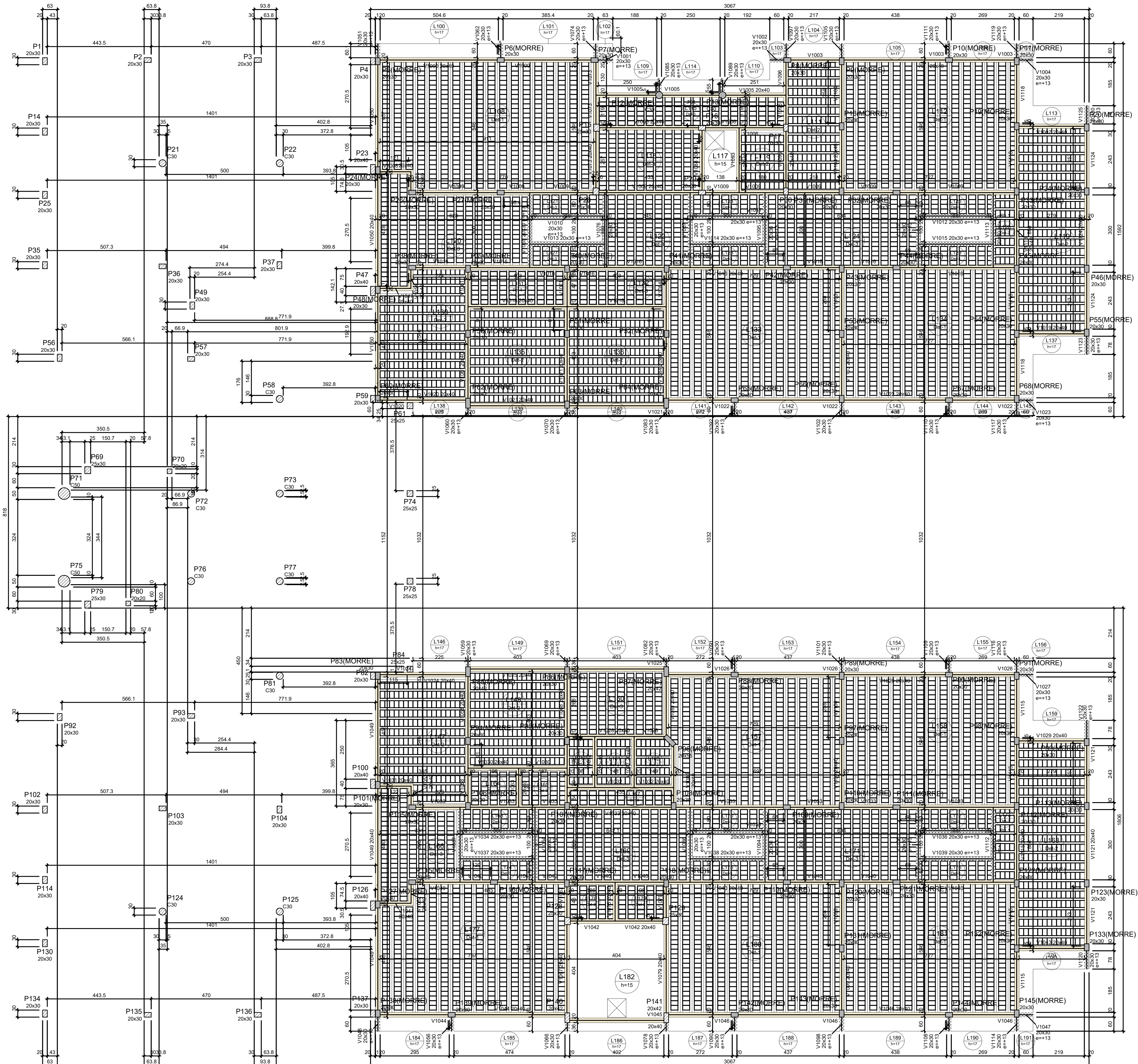
Forma do pavimento Cobertura - blocos de salas (Nível 425)
