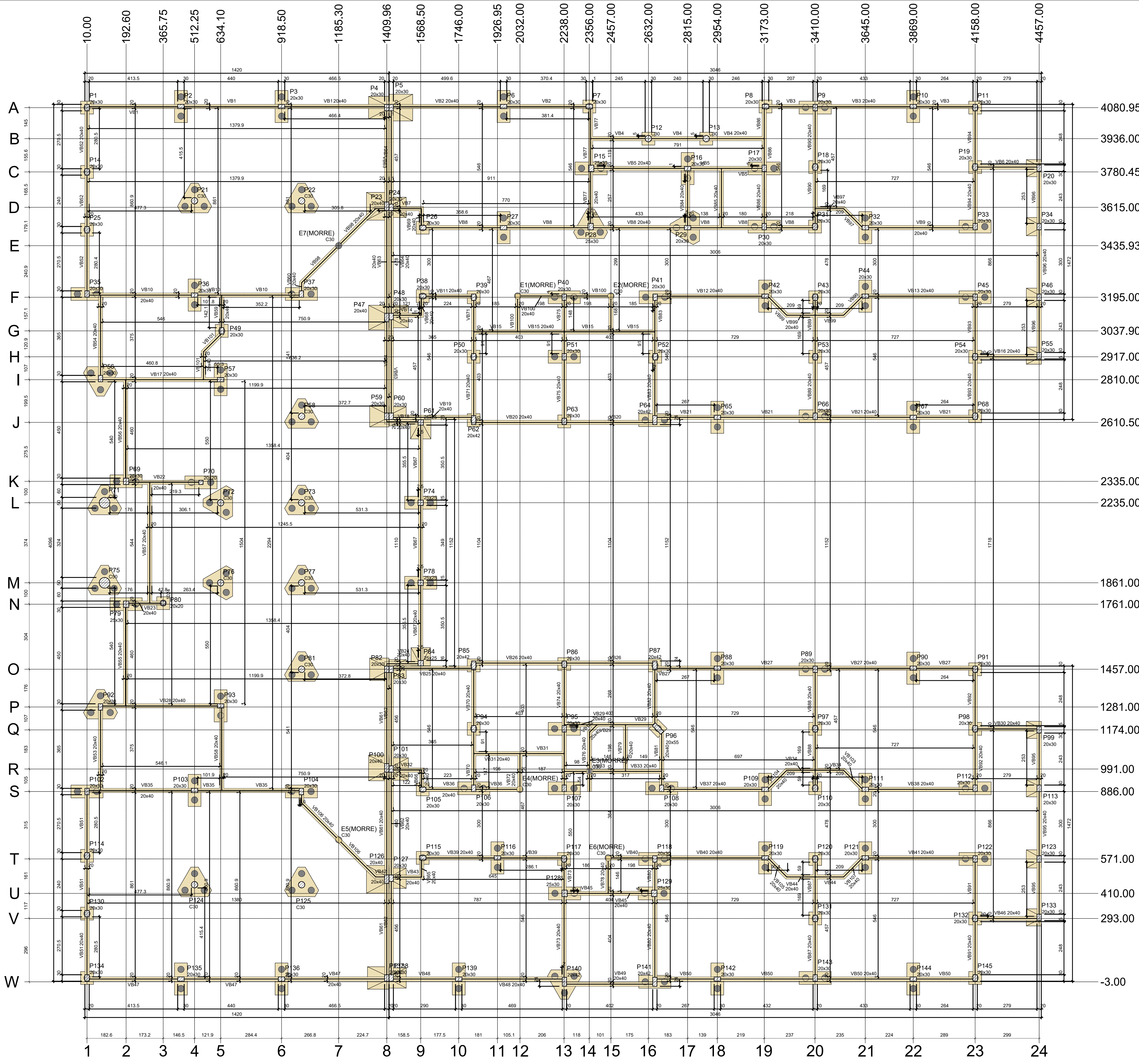
Forma do pavimento Fundação Têrreo
