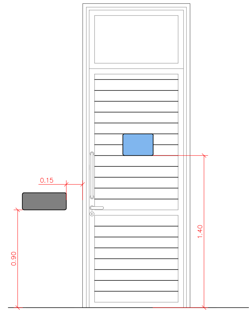
PLACAS DE INFORMAÇÃO TÁTIL SIMPLES E DUPLA - NBR 9050 ESC. - 1/5
