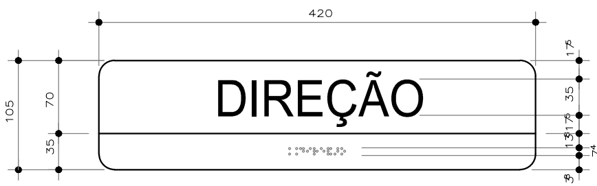
PLACAS DE INFORMAÇÃO TÁTIL SIMPLES E DUPLA - NBR 9050 ESC. - 1/5
